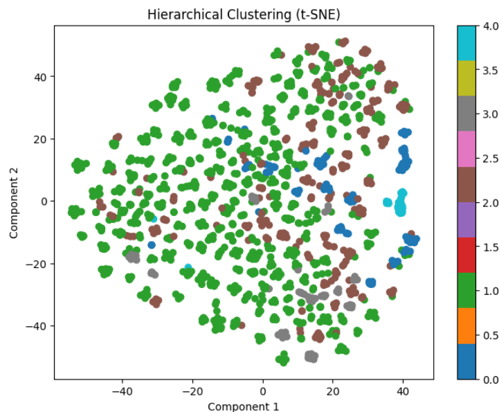
Слика 5.4: t-SNE визуелизација резултата хијерархијског кластеровања ( n = 2000 )
