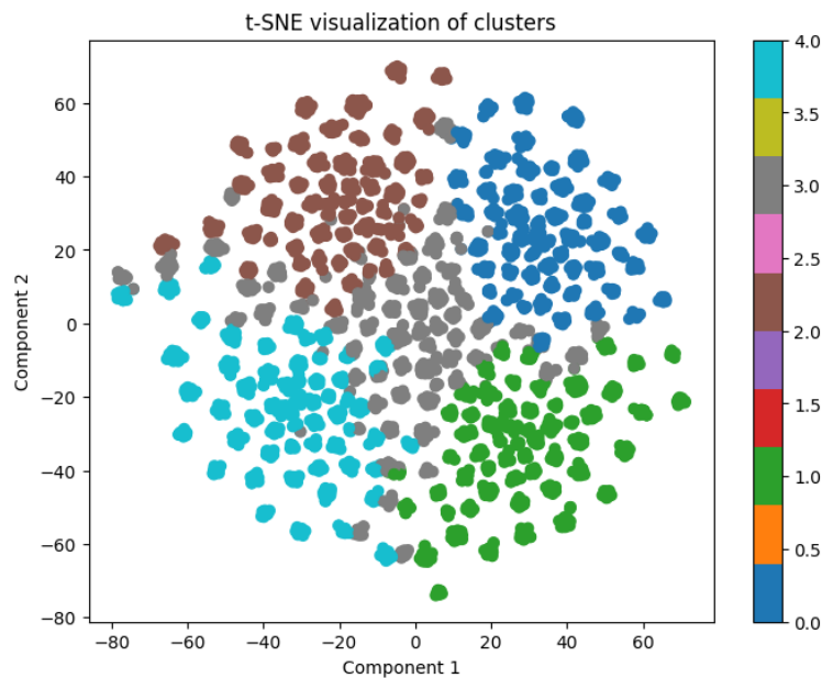
Слика 5.1: Визуелизација кластера добијених K-Means алгоритмом применом t-SNE редукције
