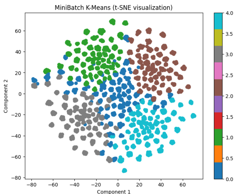
Слика 5.2: Дводимензионална t-SNE пројекција кластера генерисаних Mini-Batch K-Means алгоритмом
