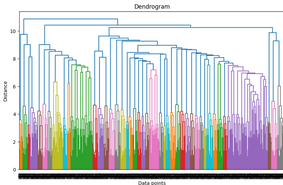
Слика 5.3: Дендрограм генерисан применом Вордове методе спајања над узорком података
