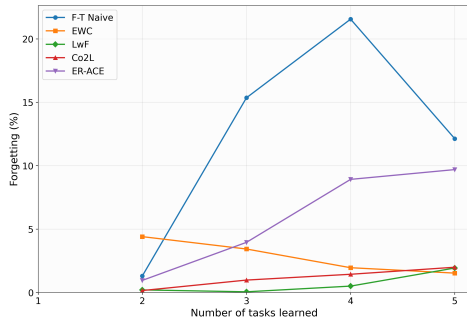
Figura 9. Olvido promedio acumulado en el escenario de incremento de tareas ( Task-IL ).
