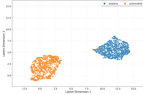
Figura 4. Estado final del espacio latente al finalizar el pre-entrenamiento (50 épocas).
