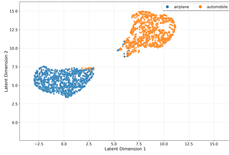
Figura 3. Evolución del espacio latente a mitad del pre-entrenamiento (25 épocas).
