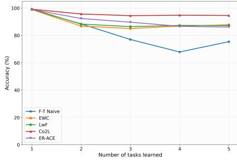
Figura 7. Evolución de la precisión promedio ( accuracy ) en el escenario Task-Incremental Learning (Task-IL) de los métodos implementados.
