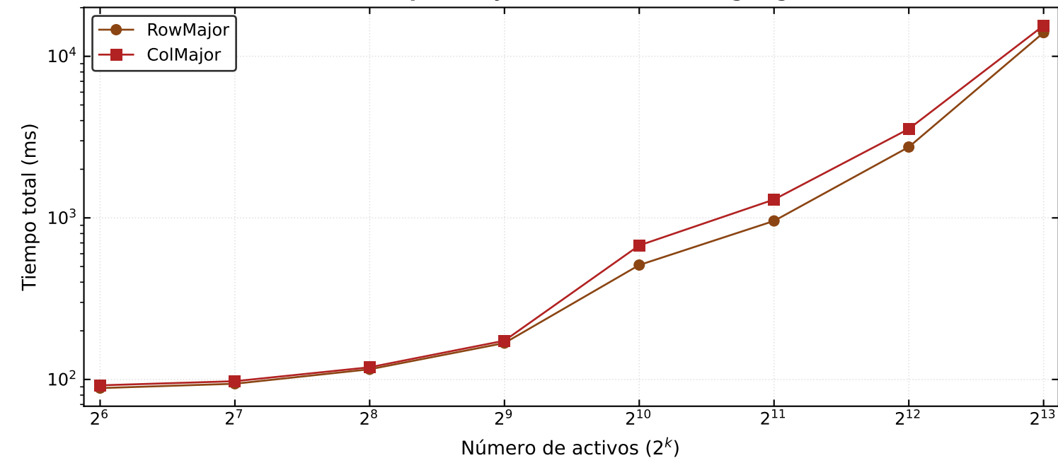
Tiempo de ejecución — escala log-log
