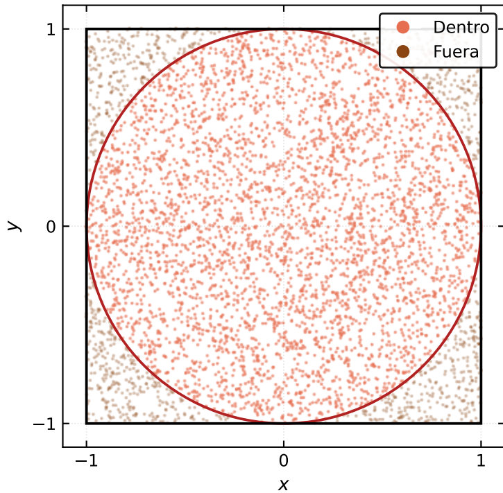
(b) Lanzamiento de N = 5000 dardos aleatorios
