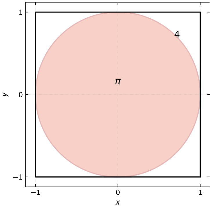
(a) Cuadrado de área 4 y círculo de área \pi
