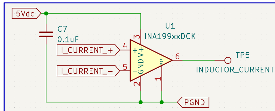
Figura 10: Medición de corriente unidireccional con INA199B2.
