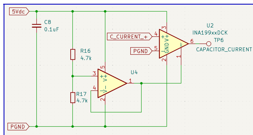
Figura 11: Medición de corriente bidireccional con INA199B2.
