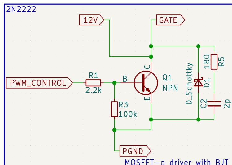
Figura 9: Transistor 2N2222 como driver de MOSFET-p.
