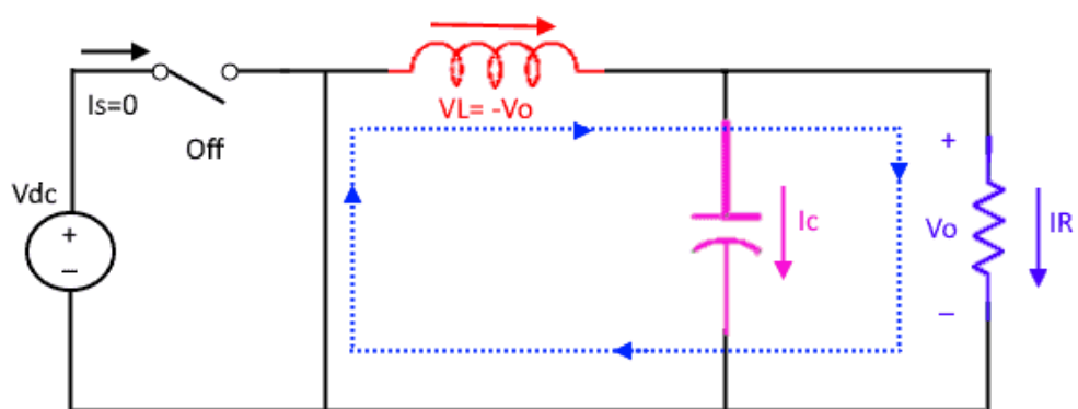
Figura 6: Interruptor en estado de no conducción.
