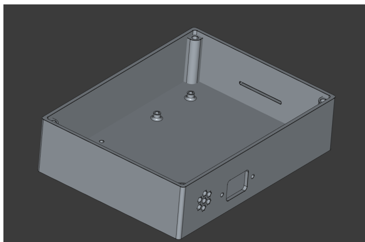
(a) Base de gabinete general.
