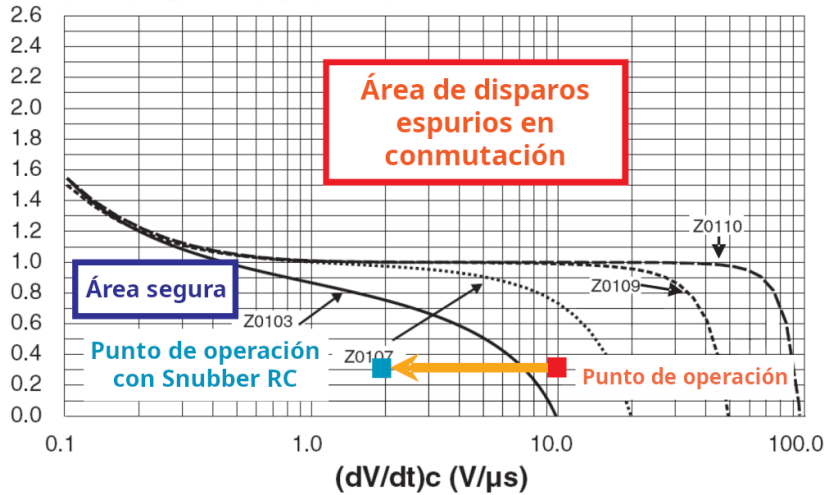
(b) Curva (dI/dt)_c según (dV/dt)_c para TRIACs Z01, con y sin red Snubber, (STMicroelectronics, 2024)
