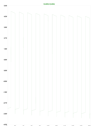
(b) Señal en la carga.
