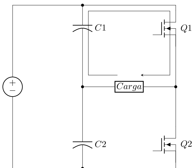
Figura 25: Conmutación 1.
