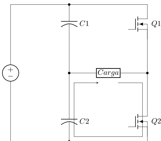
Figura 26: Conmutación 2.
