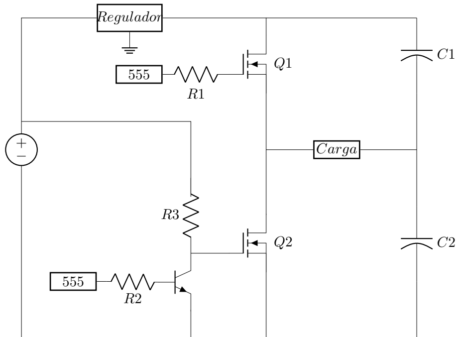
Figura 2: Circuito de inversor medio puente.
