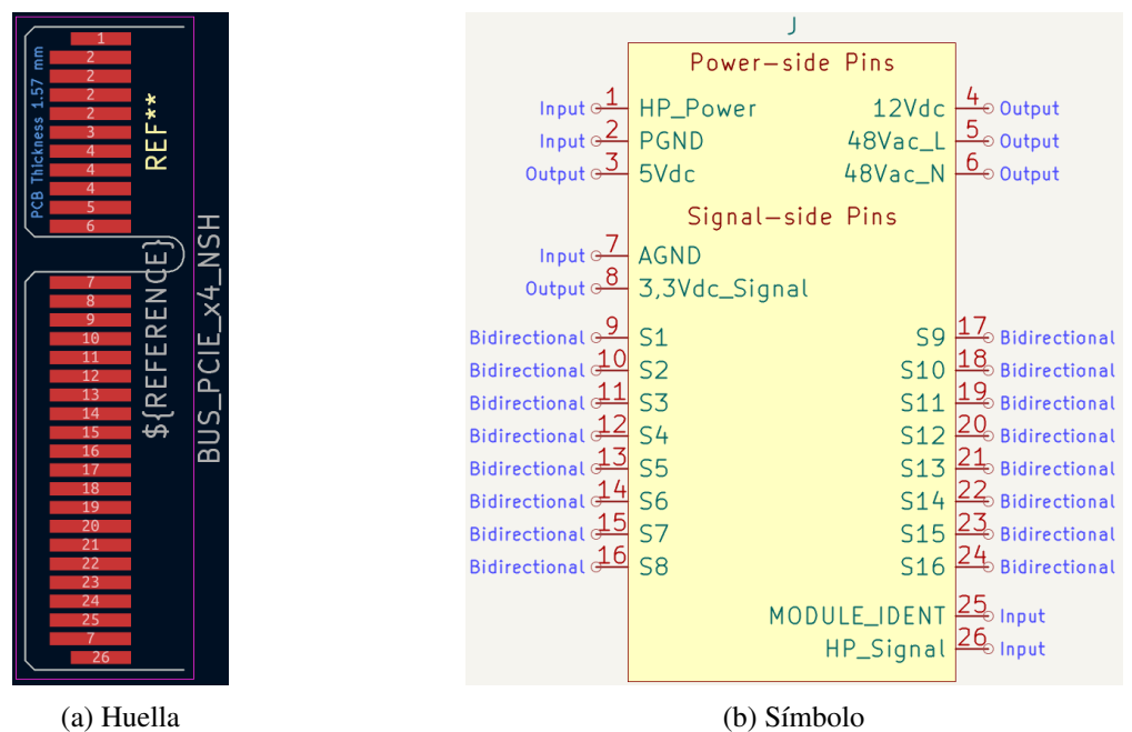
Figura 38: Símbolo y huella del conector PCIe x4
