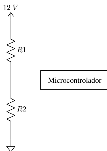
Figura 7: Divisor de tensión genérico.
