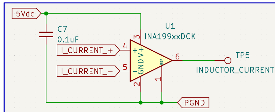
Figura 10: Medición de corriente unidireccional con INA199B2.
