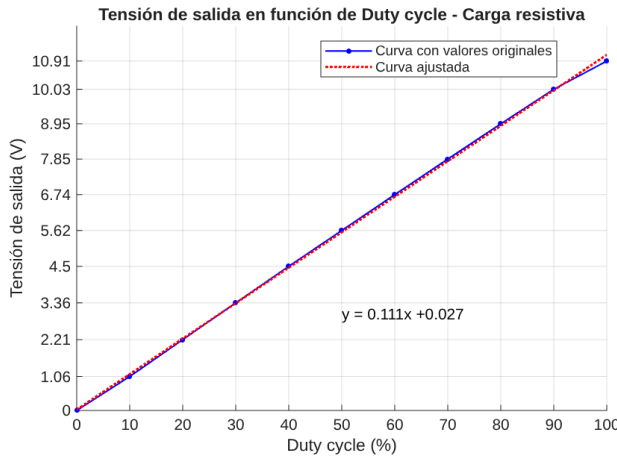
(a) Con carga resistiva.
