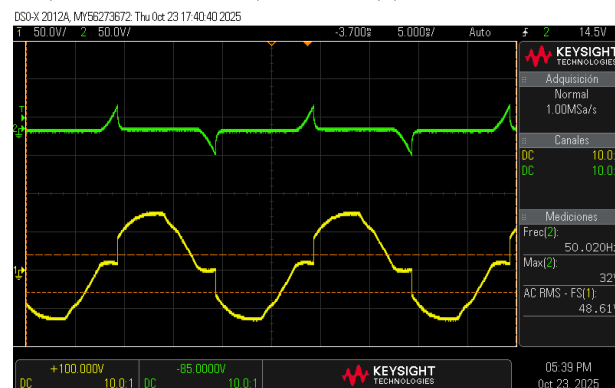
(c) Potenciómetro al máximo(resistencia mínima).
