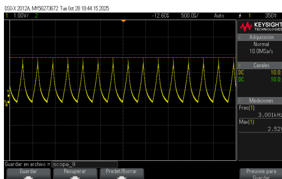
(a) modo de conducción continua (CCM).
