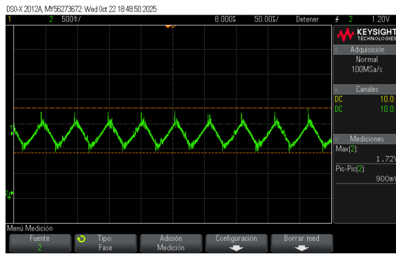
(a) Inductor.
