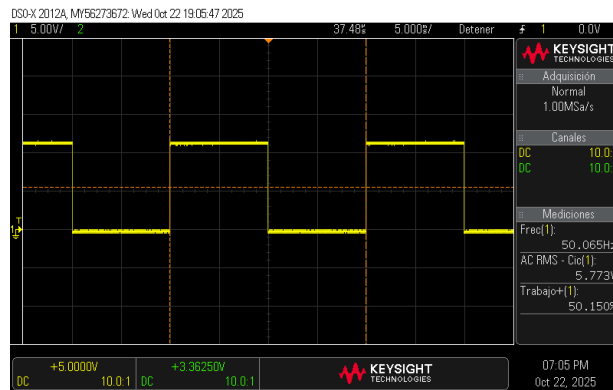
(a) 50 Hz.
