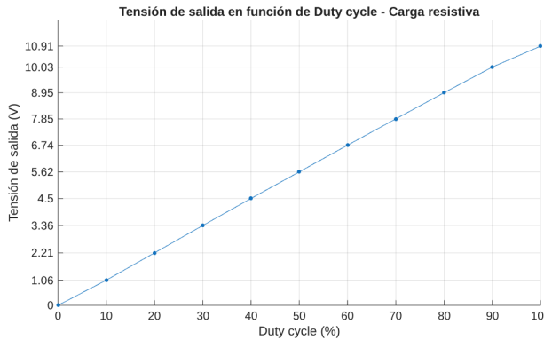
(a) Con carga resistiva.
