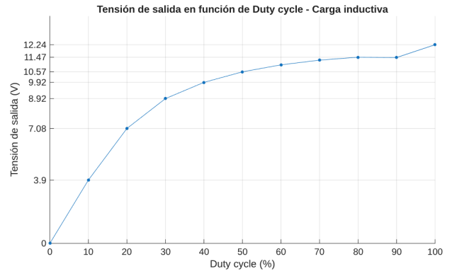
(b) Con carga inductiva.
