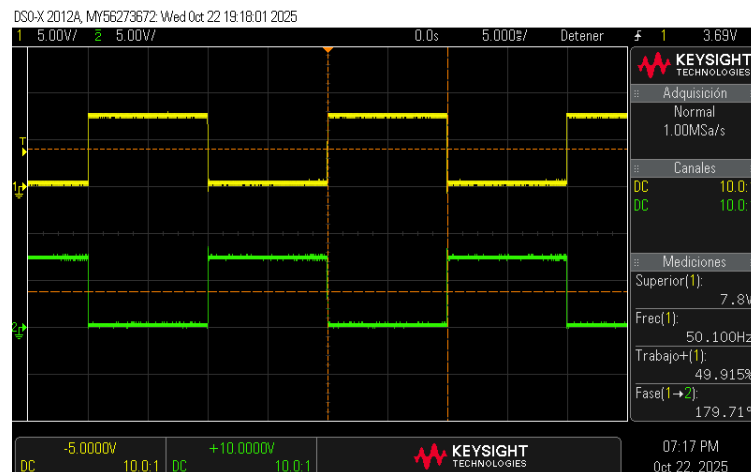
Figura 61: Tensión drenador-surtidor de los MOSFETs.
