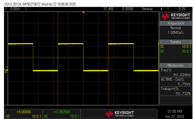
(b) 60 Hz.
