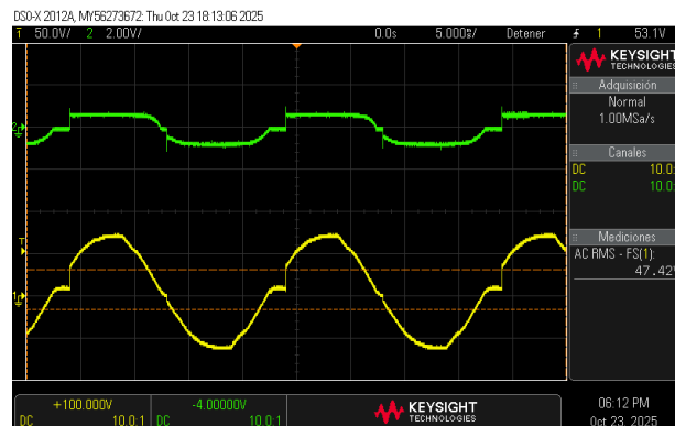
(c) Tiempo de espera máximo (9,2 ms).
