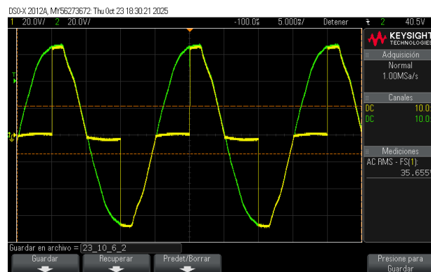
Figura 59: Potenciómetro al mínimo (resistencia máxima).
