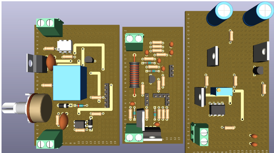
Figura 41: Vista frontal de los modelos 3D de las placas experimentales perforadas. De izquierda a derecha: módulo recortador de onda, módulo convertidor Buck, módulo inversor de onda cuadrada
