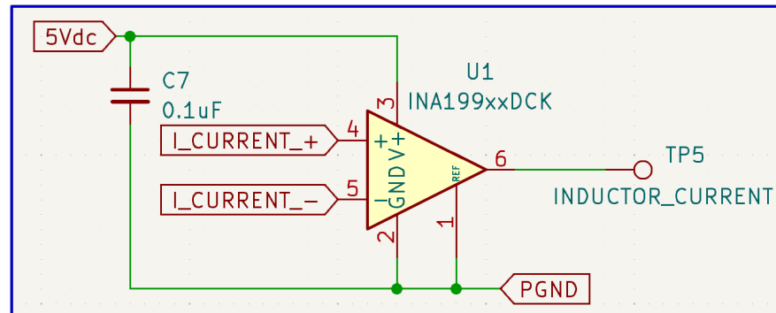
Figura 17: Medición de corriente unidireccional con INA199B2.
