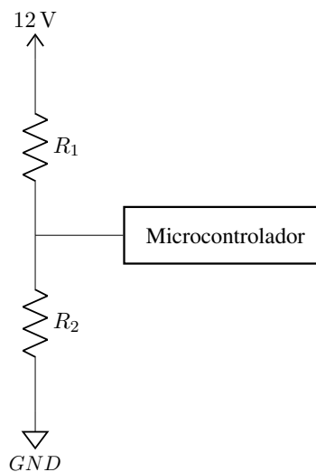
Figura 14: Divisor de tensión genérico.
