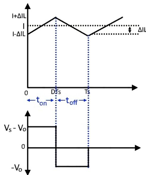
Figura 10: Tensión y corriente en el inductor. Fuente: (Electrical Technology, 2020)
