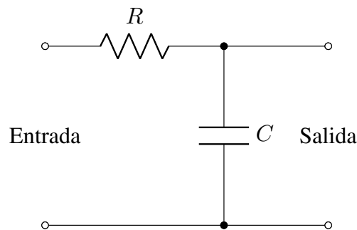
Figura 15: Filtro pasa-bajos genérico.
