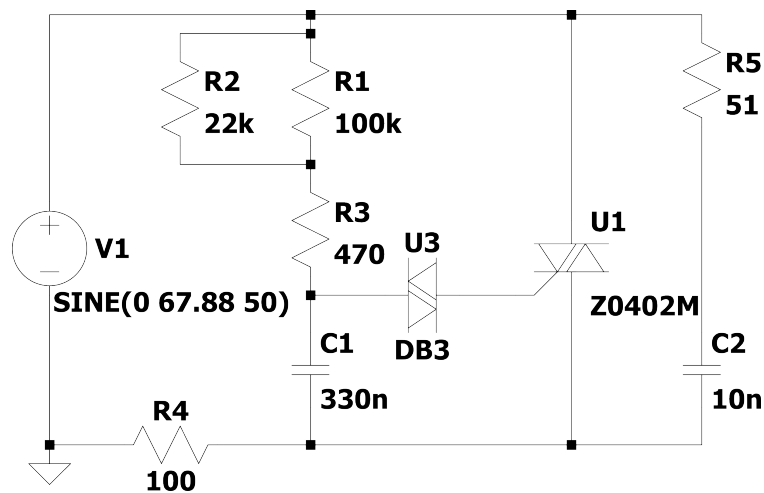
Figura 30: Circuito en LTSpice 6
