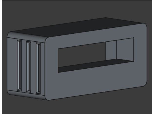
Figura 2: Carcasa para conector PCIe x4.
