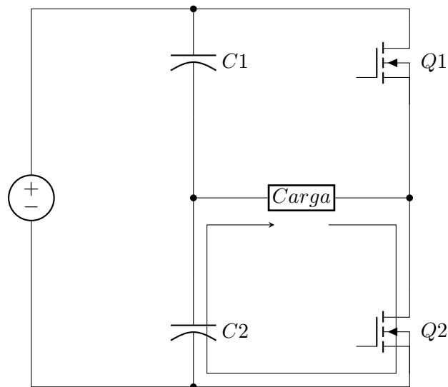
Figura 36: Conmutación 2.
