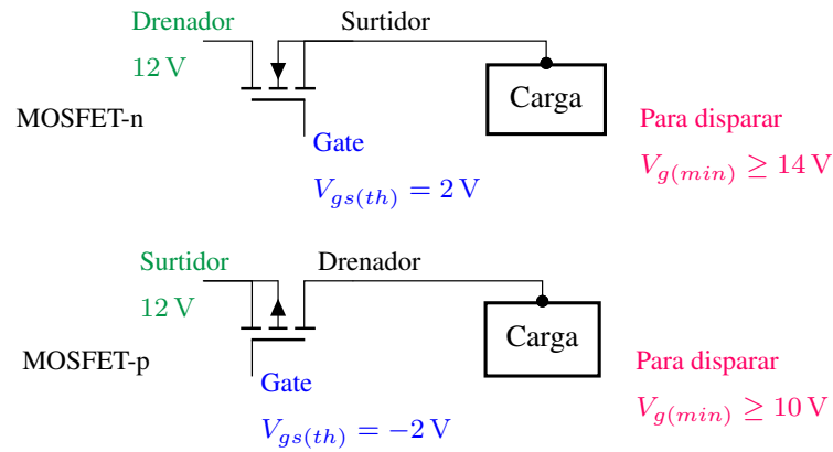
Figura 6: MOSFET-n vs MOSFET-p.
