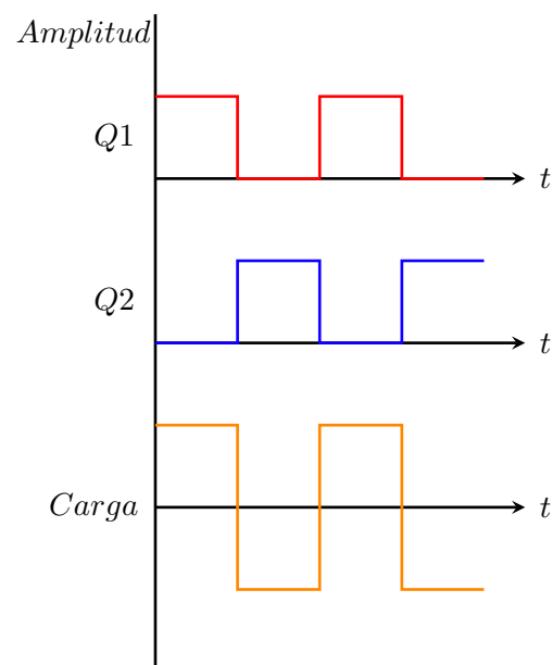
Figura 37: Forma de onda.
