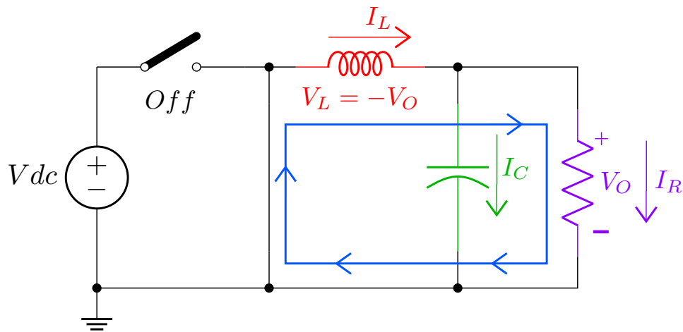
Figura 11: Interruptor en estado de no conducción.
