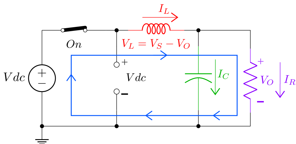
Figura 9: Interruptor en conducción.
