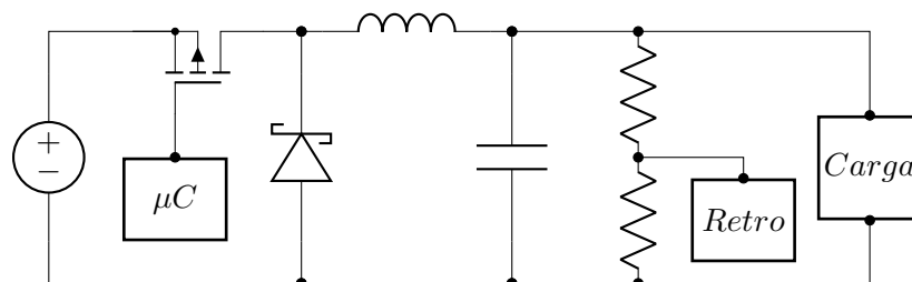
Figura 5: Circuito básico del convertidor Buck.
