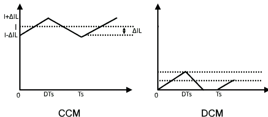
Figura 8: Modos de funcionamiento. Fuente: (Electrical Technology, 2020)
