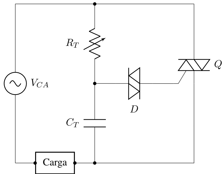
Figura 23: Circuito básico de control de fase.
