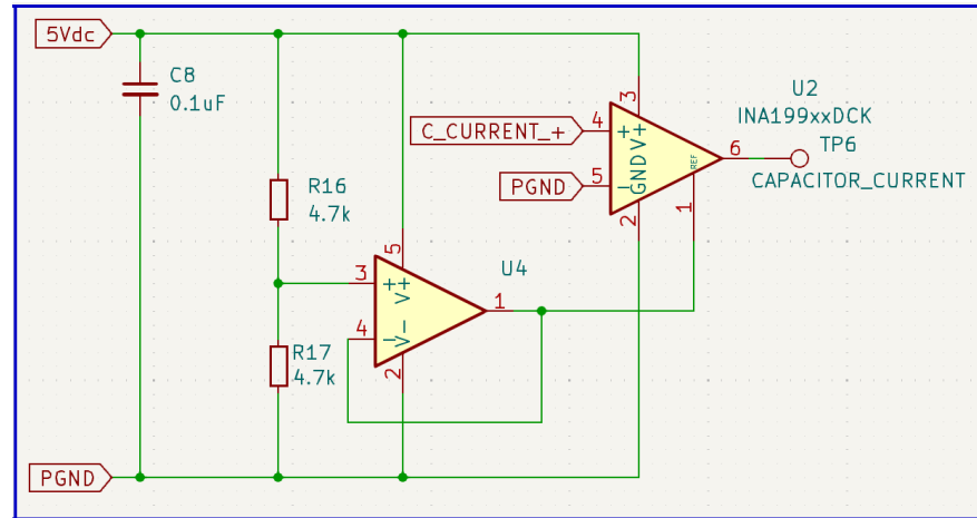
Figura 18: Medición de corriente bidireccional con INA199B2.
