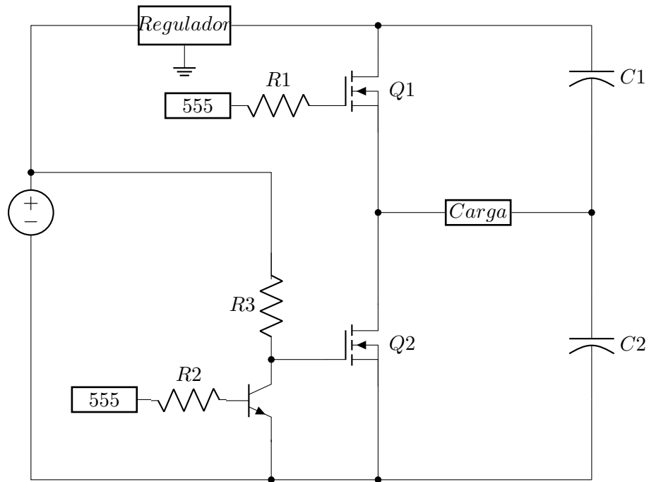
Figura 33: Circuito de inversor medio puente.
