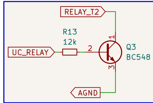
Figura 19: Circuito driver para relé.
