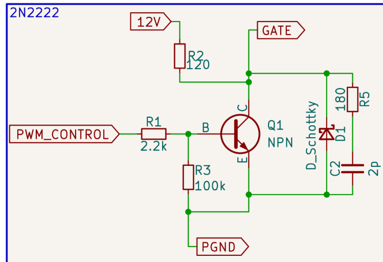
Figura 17: Transistor 2N2222 como driver de MOSFET-p.
