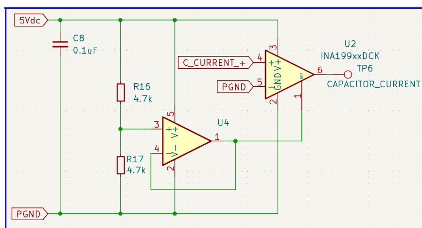
Figura 12: Medición de corriente bidireccional con INA199B2.
