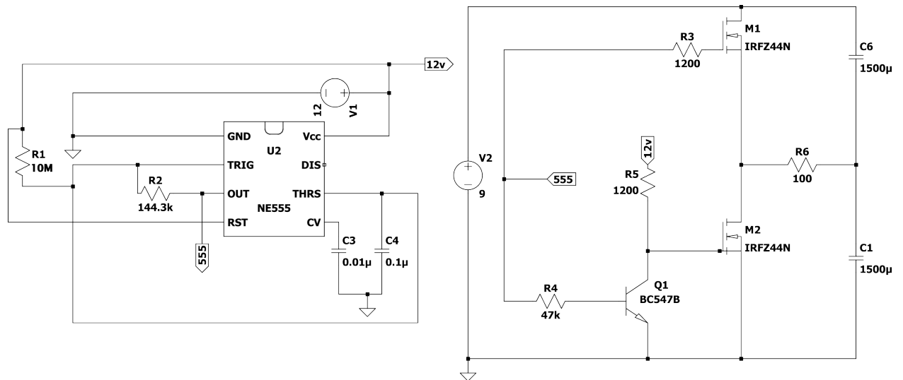
Figura 33: Circuito en LTSpice.
