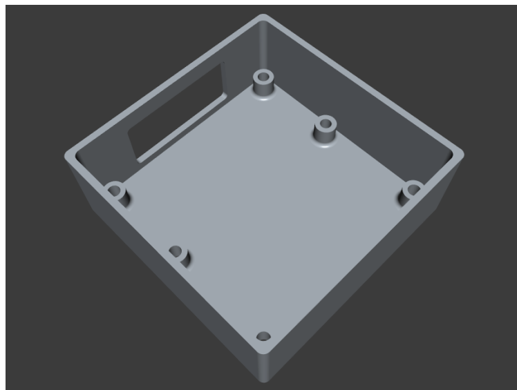
Figura 40: Gabinete individual.
