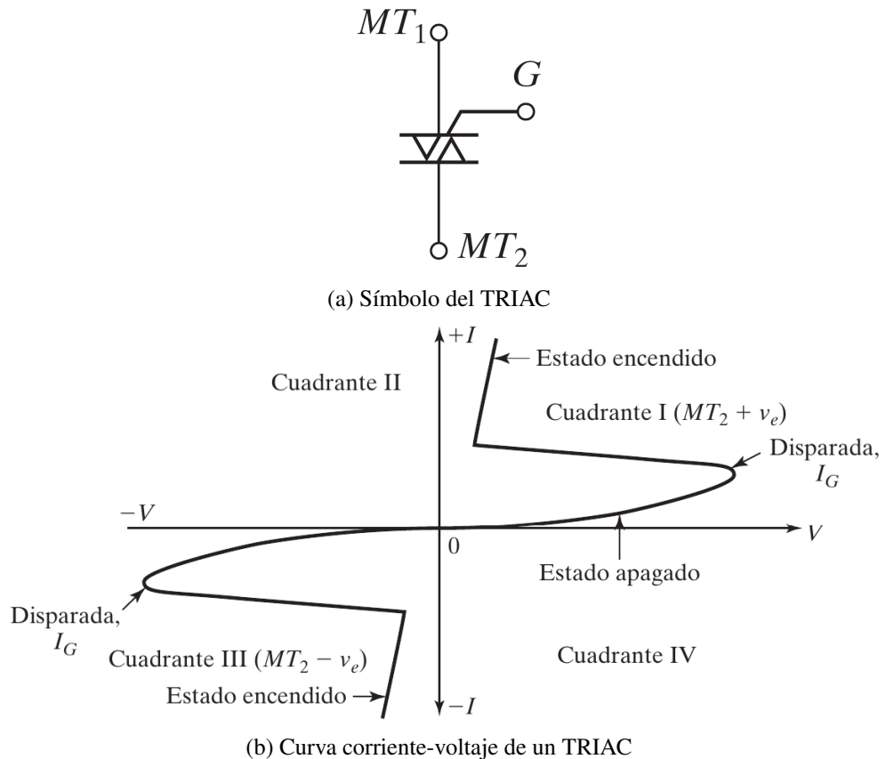
Figura 15: Características del TRIAC. Fuente: (Rashid, 2015)
