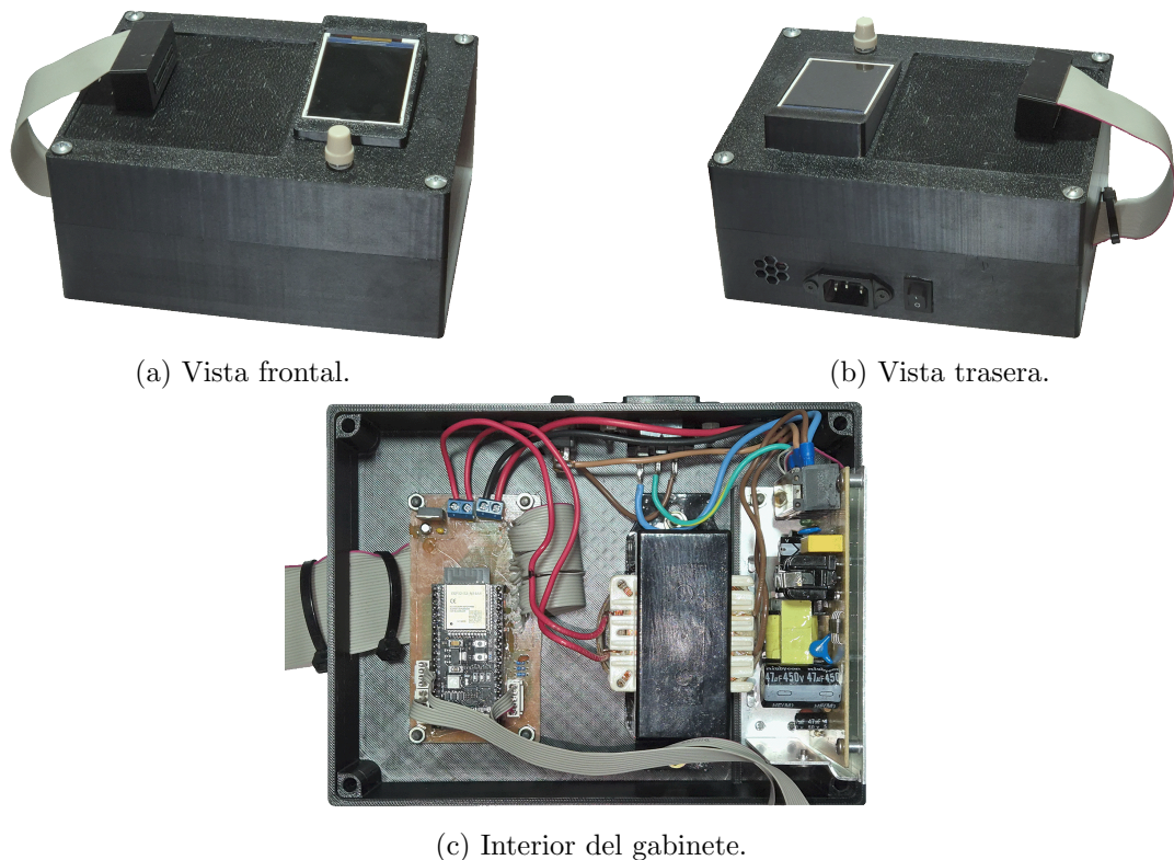
Figura 51: Gabinete central del sistema.
