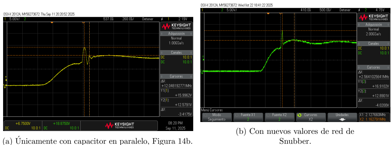
Figura 16: Resultados en transistor 2N2222 en circuito real
