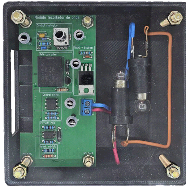
Figura 59: Gabinete del módulo recortador de onda.
