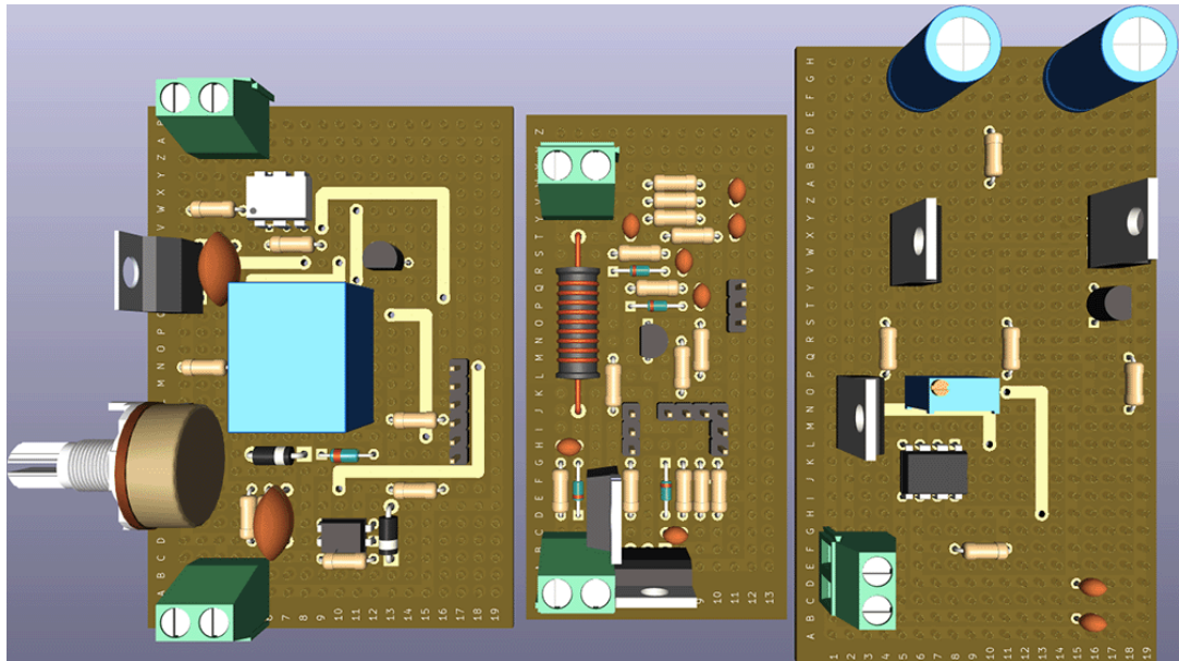
Figura 44: Vista frontal de los modelos 3D de las placas experimentales perforadas. De izquierda a derecha: módulo recortador de onda, módulo convertidor Buck, módulo inversor de onda cuadrada
