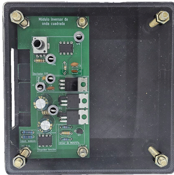
Figura 64: Gabinete del módulo inversor de onda cuadrada.
