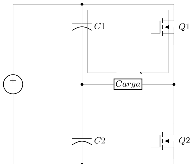
Figura 38: Conmutación 1.
