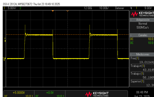
Figura 53: Tensión de gate del transistor IRF9540.
