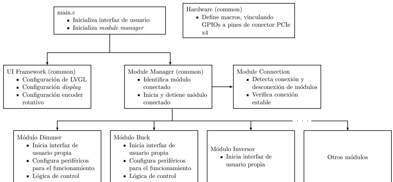
Figura 49: Estructura del código implementado
