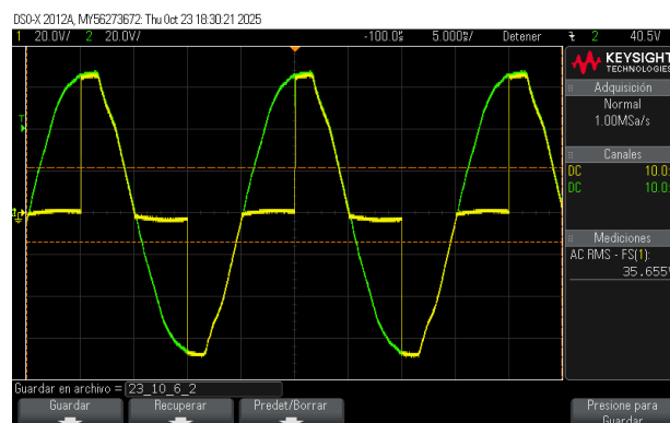
Figura 60: Recortador de onda en control analógico. Señal verde: tensión de entrada. Señal amarilla: tensión aplicada en la carga
