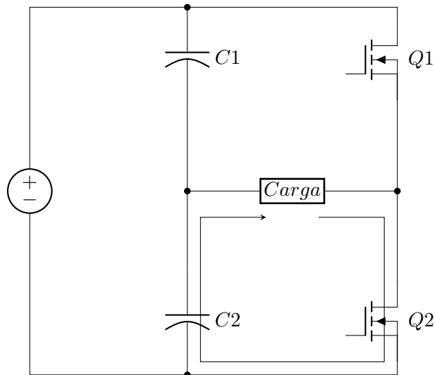
Figura 39: Conmutación 2.
