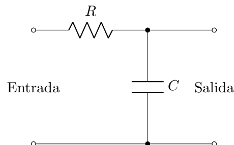
Figura 18: Filtro pasa-bajos genérico.
