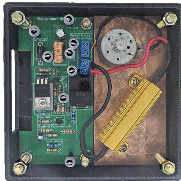
Figura 52: Gabinete del módulo convertidor reductor.
