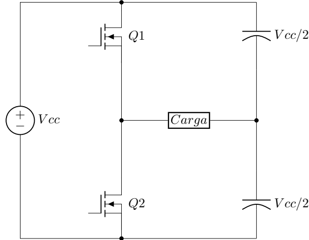
Figura 41: Inversor medio puente con control por 555
