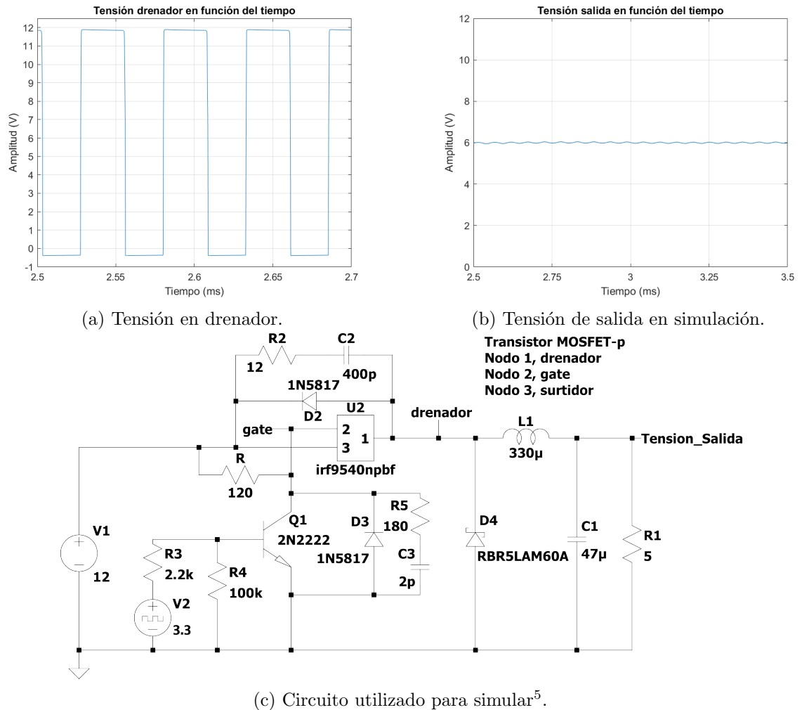
Figura 23: Resultados de la simulación con un ciclo de trabajo del 50 %.
