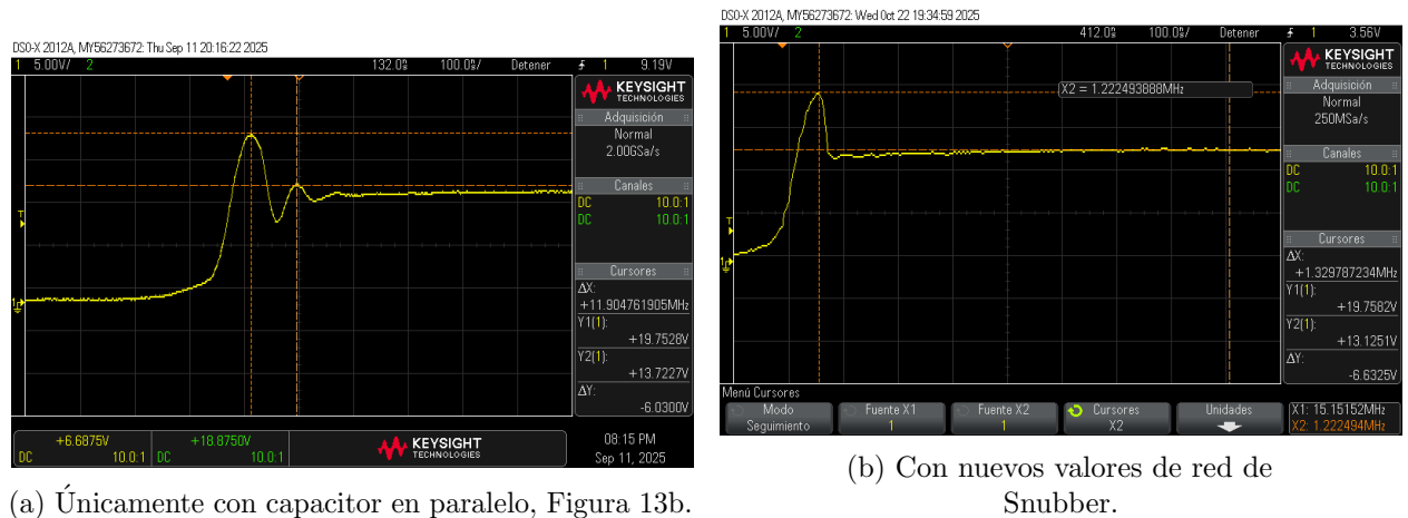
Figura 15: Resultados en transistor IRF9540 en circuito real
