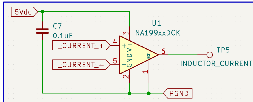
Figura 20: Medición de corriente unidireccional con INA199B2.
