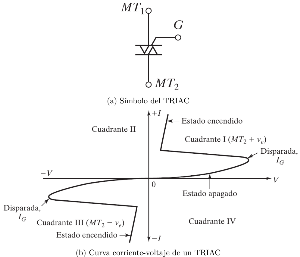
Figura 24: Características del TRIAC.
