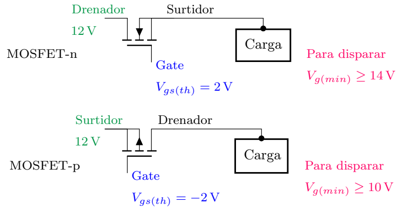
Figura 7: MOSFET-n vs MOSFET-p.
