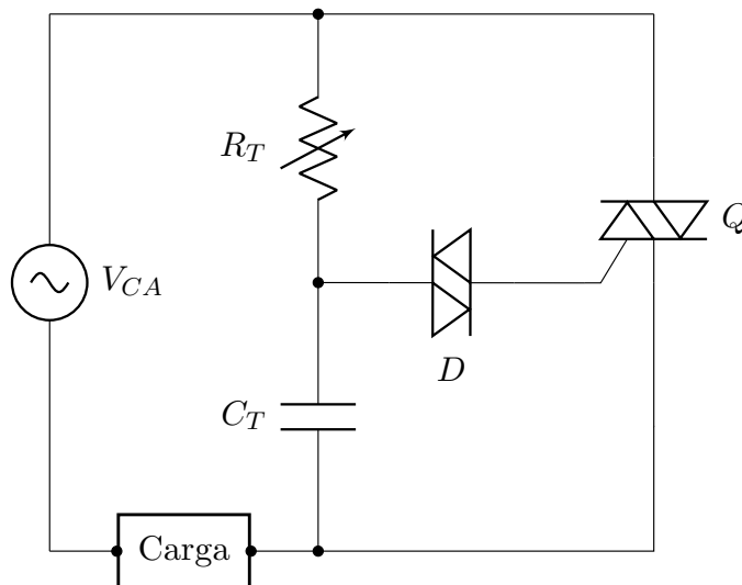
Figura 26: Circuito básico de control de fase.
