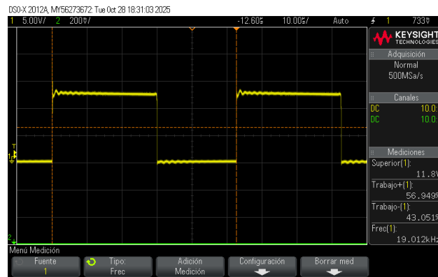
Figura 54: Tensión conmutada en drenador del transistor IRF9540.
