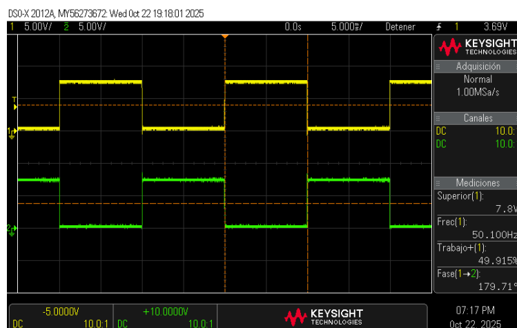
Figura 66: Tensión drenador-surtidor de los MOSFETs. En amarillo, Q1 y en verde, Q2.
