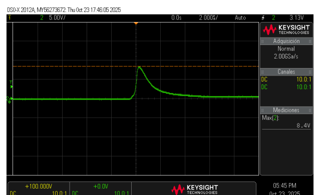
(b) Vista ampliada del pulso en la tensión de gate del TRIAC.
