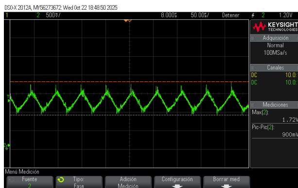
(a) Inductor.
