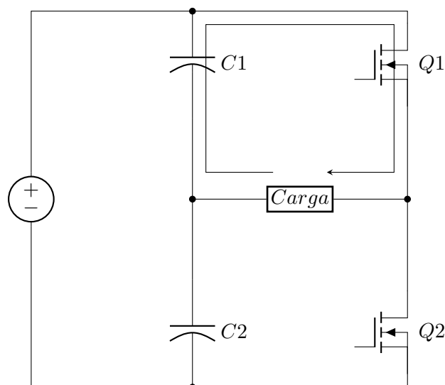
Figura 25: Conmutación 1.
