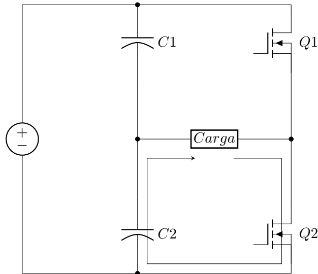
Figura 26: Conmutación 2.
