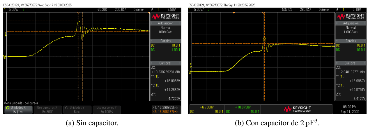
Figura 9: Resultados en transistor 2N2222 en circuito real
