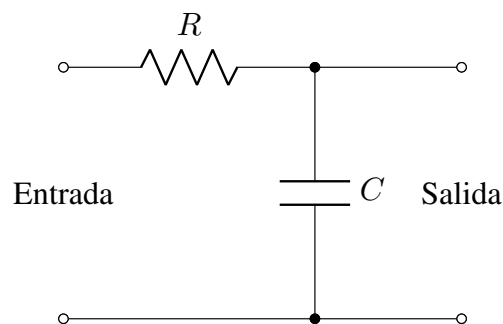
Figura 16: Filtro pasa-bajos genérico.
