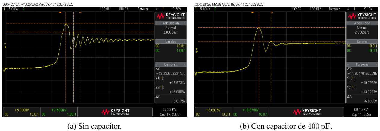
Figura 13: Resultados en transistor IRF9540 en circuito real
