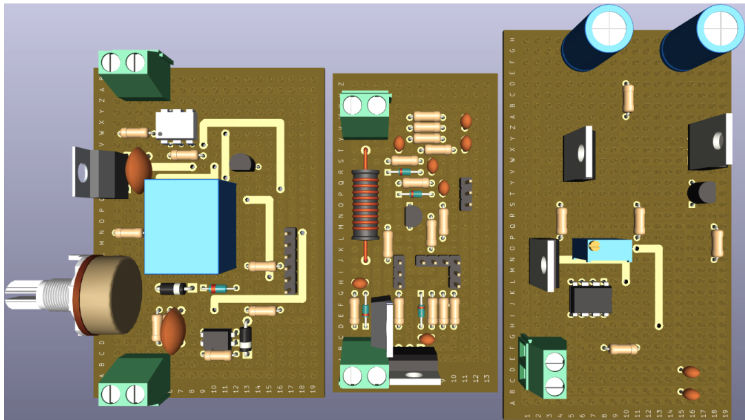
Figura 42: Vista frontal de los modelos 3D de las placas experimentales perforadas. De izquierda a derecha: módulo recortador de onda, módulo convertidor Buck, módulo inversor de onda cuadrada
