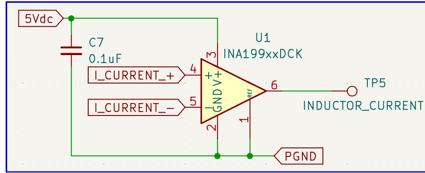
Figura 18: Medición de corriente unidireccional con INA199B2.
