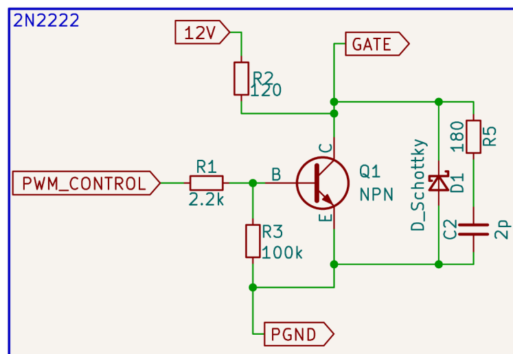
Figura 17: Transistor 2N2222 como driver de MOSFET-p.
