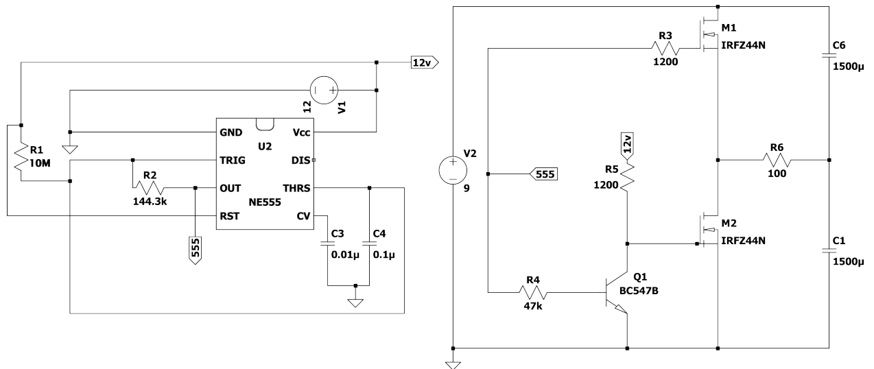
Figura 40: Circuito en LTspice.
