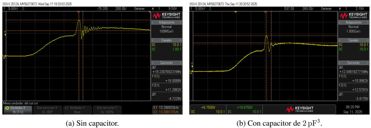
Figura 14: Resultados en transistor 2N2222 en circuito real
