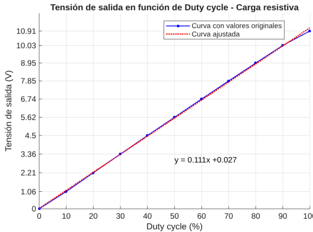
(a) Con carga resistiva.
