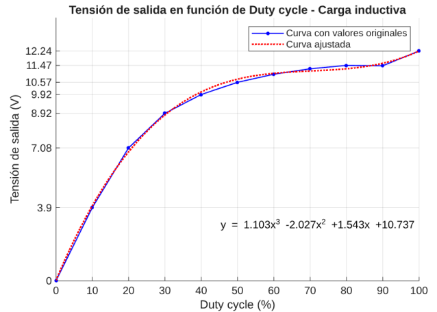
(b) Con carga inductiva.
