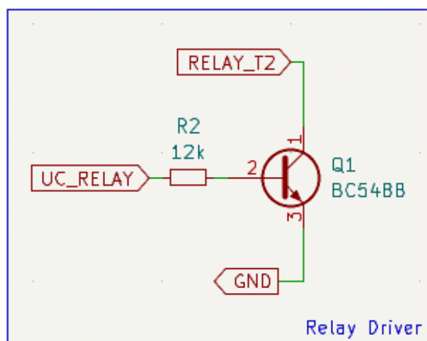
Figura 8: Driver de relé.
