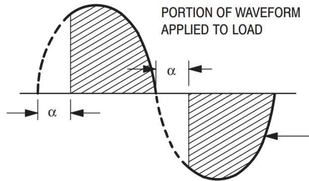
Figura 3: Control de fase de onda de corriente alterna.
