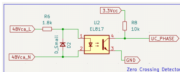
Figura 6: Circuito ZCD.
