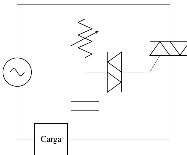
Figura 1: Circuito básico recortador de onda analógico.
