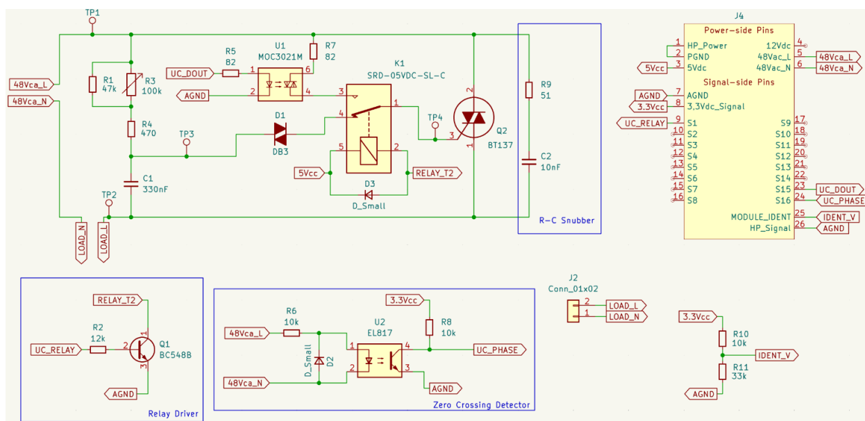
Figura 2: Circuito completo del módulo recortador de onda.
