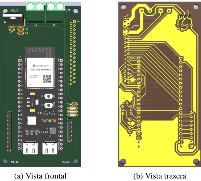
Figura 32: Modelo 3D de las PCB general del control del gabinete.
