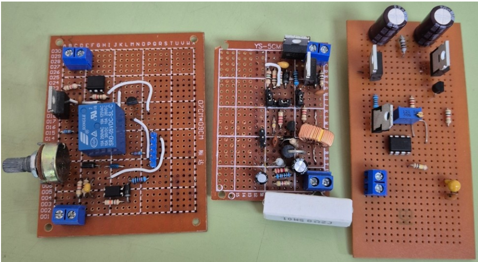
Figura 29: Placas experimentales perforadas. De izquierda a derecha: prototipos de módulo recortador de onda, módulo convertidor Buck, módulo inversor de onda cuadrada.
