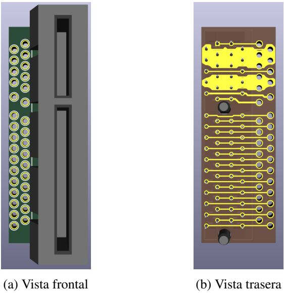
Figura 33: Modelo 3D de la mini-PCB para el conector PCIe X4.
