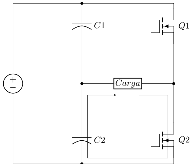
Figura 27: Conmutación 2.
