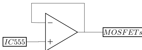
Figura 25: Seguidor de tensión.
