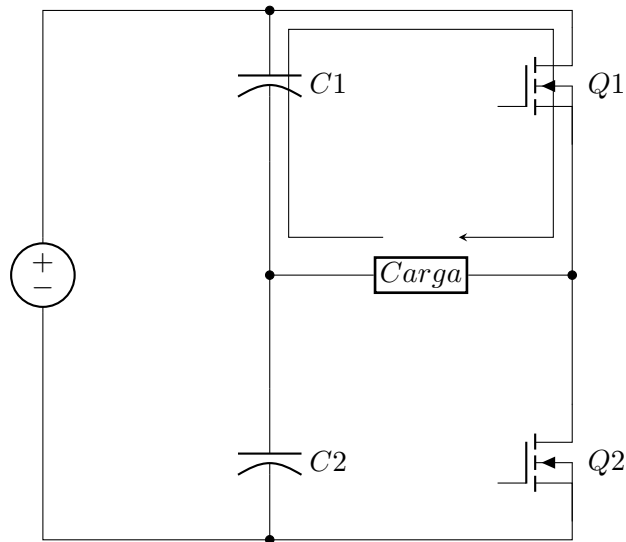
Figura 26: Conmutación 1.
