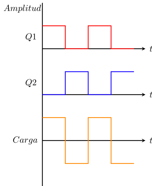
Figura 28: Forma de onda.
