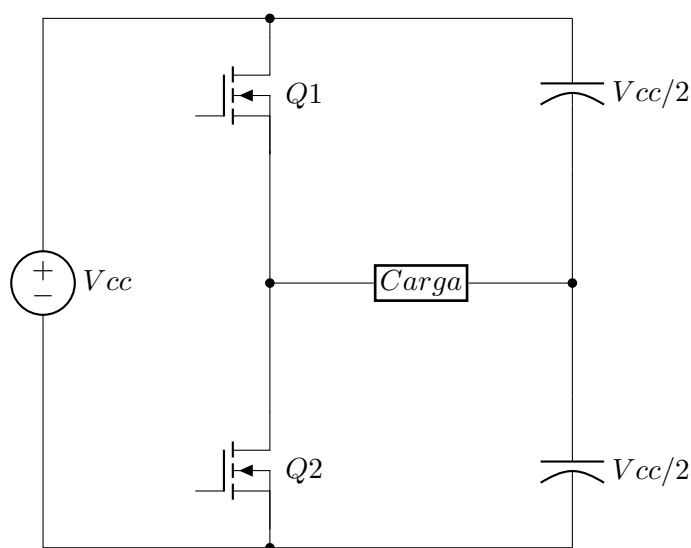
Figura 29: Inversor medio puente con control por 555
