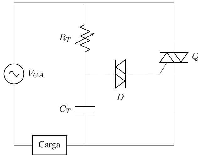
Figura 3: Circuito básico de control de fase.
