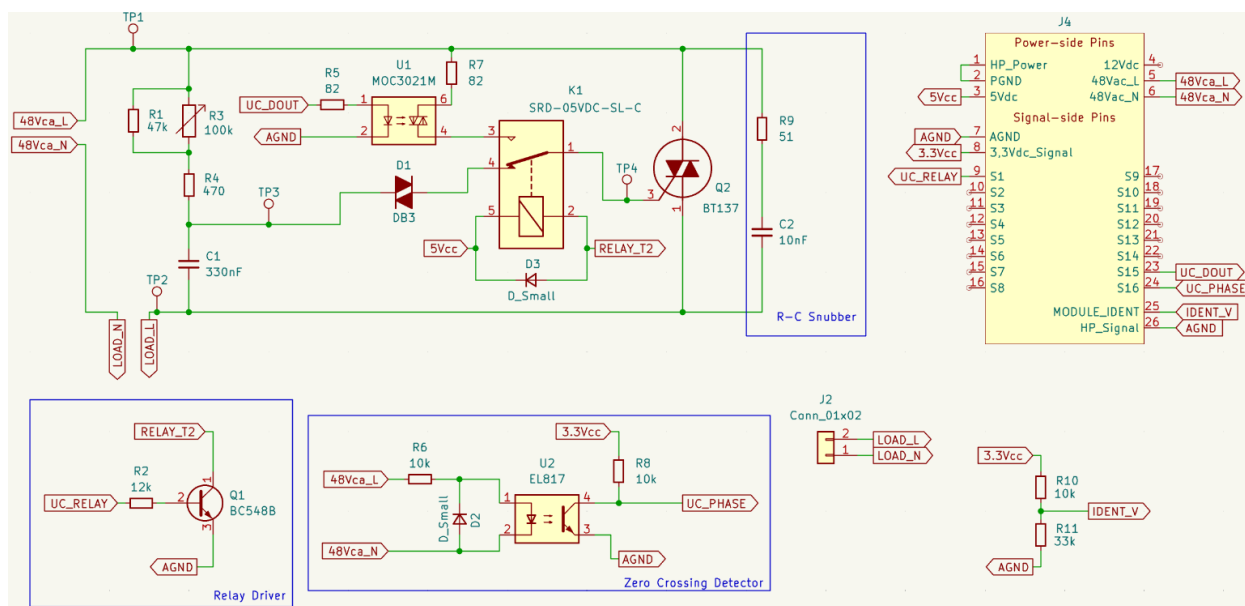
Figura 6: Circuito completo del módulo recortador de onda.
