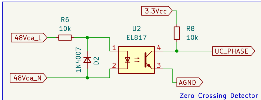
Figura 5: Circuito detector de cruce por zero.
