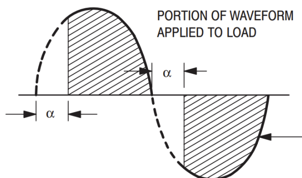
Figura 2: Control de fase de onda de corriente alterna. REFERENCIA Thyristor Theory and Design Considerations
