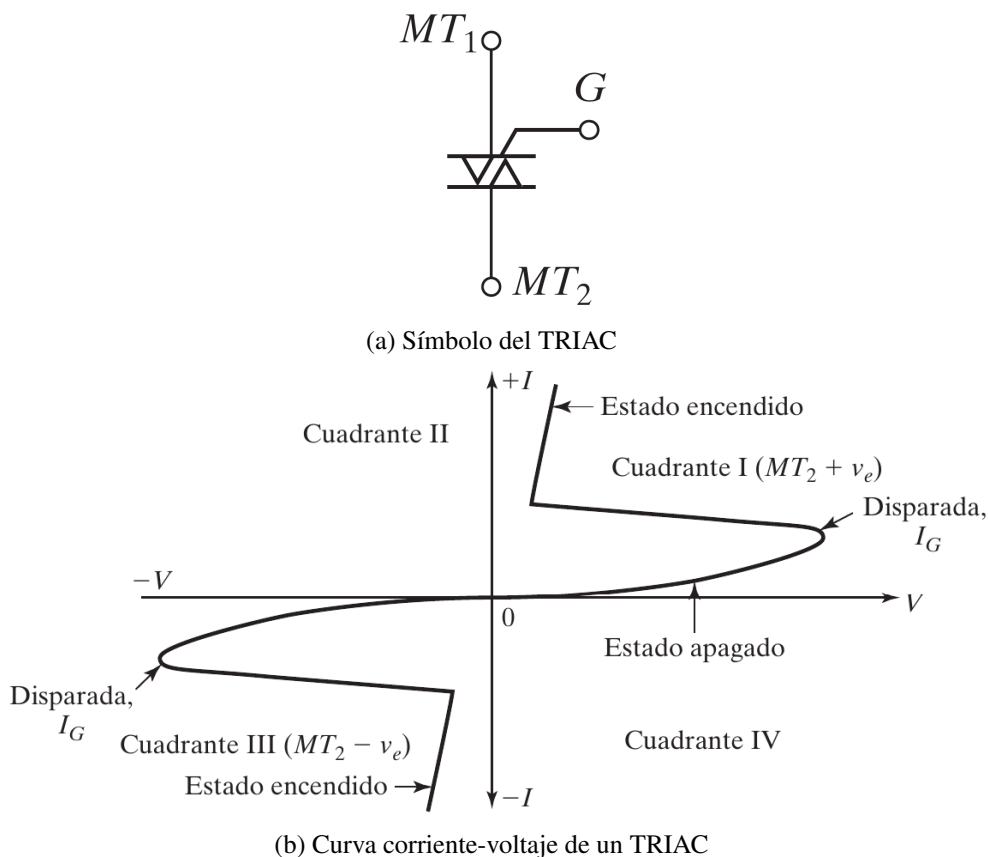
Figura 1: Características del TRIAC REFERENCIA RASHID ESPAÑOL
