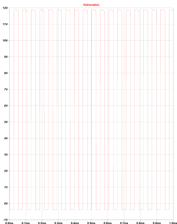
(a) Tensión en drenador de transistor de conmutación.
