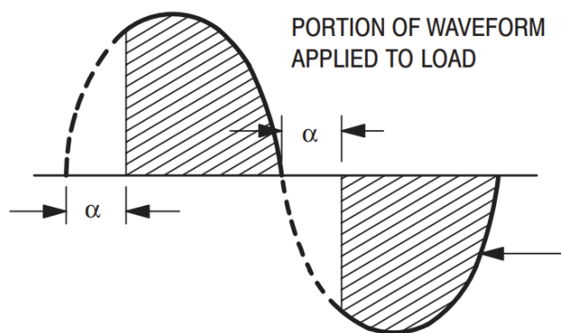
Figura 5: Control de fase de onda de corriente alterna.
