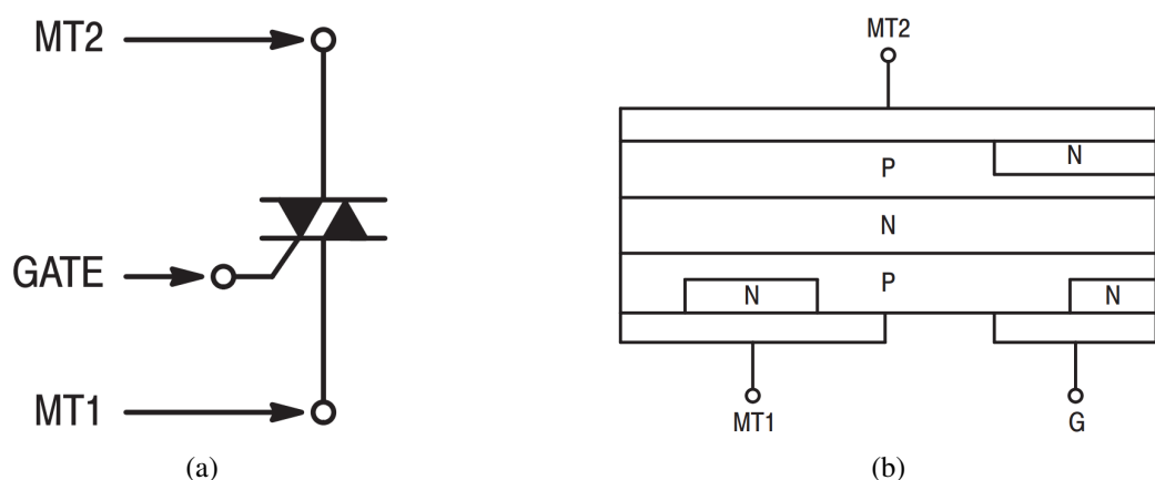
Figura 1: Símbolo y estructura del TRIAC REFERENCIA Thyristor Theory and Design Considerations
