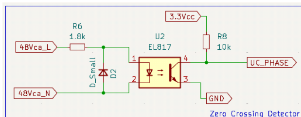
Figura 8: Circuito ZCD.
