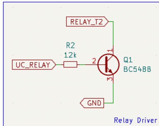
Figura 10: Driver de relé.
