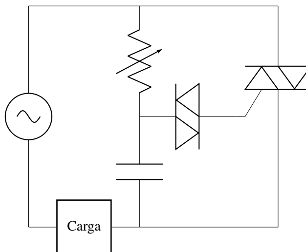
Figura 3: Circuito básico recortador de onda analógico.
