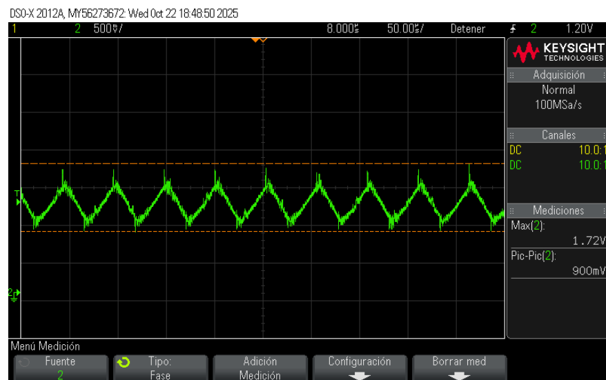
Figura 53: Corriente por el inductor.
