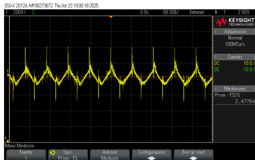
Figura 54: Corriente por el capacitor de salida.
