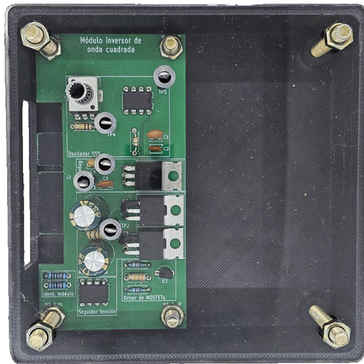
Figura 64: Gabinete del módulo inversor de onda cuadrada.
