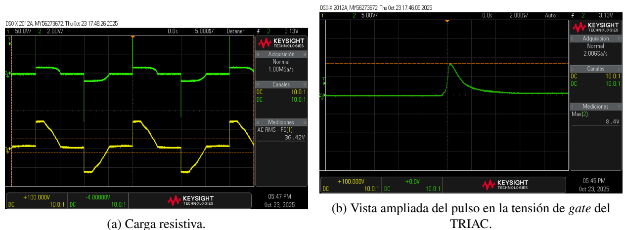
Figura 62: Recortador de onda funcionando en modo analógico. Señal verde: tensión de gate del TRIAC. Señal amarilla: tensión aplicada en la carga.
