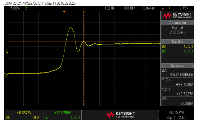
(b) Con capacitor de 400 pF.
