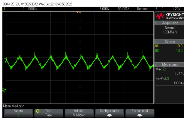
(a) Inductor.
