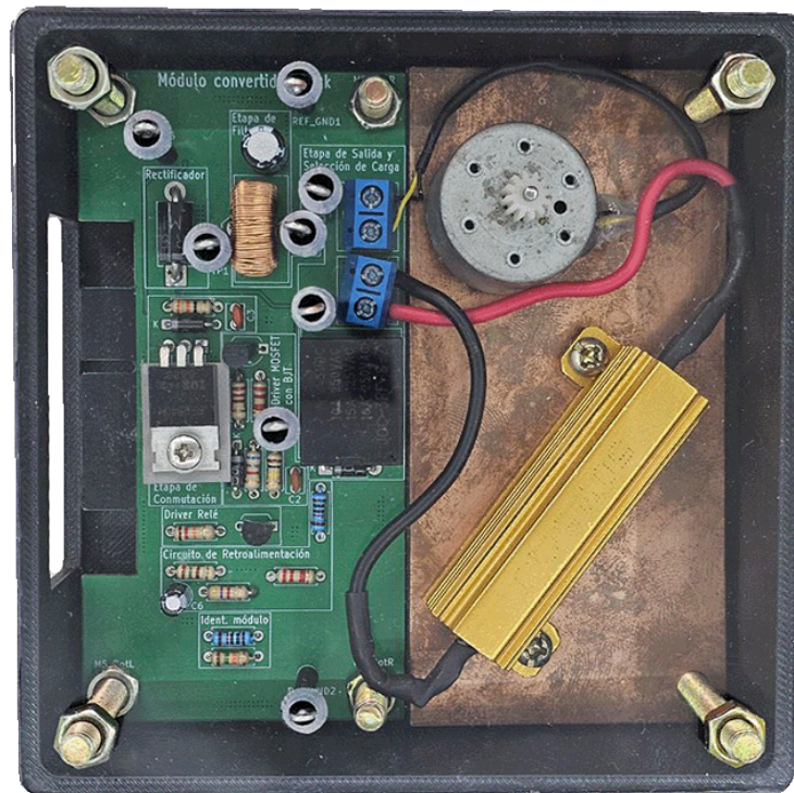
Figura 52: Gabinete del módulo convertidor reductor.
