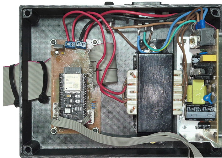
(c) Interior del gabinete.
