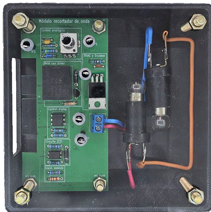
Figura 59: Gabinete del módulo recortador de onda.
