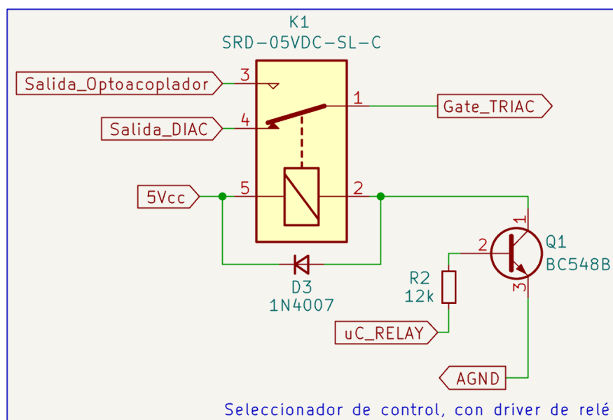
Figura 22: Circuito seleccionador de control analógico-digital.
