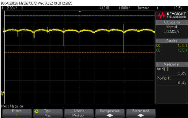
(a) Con carga inductiva.
