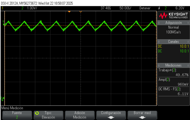
(b) Con carga resistiva.
