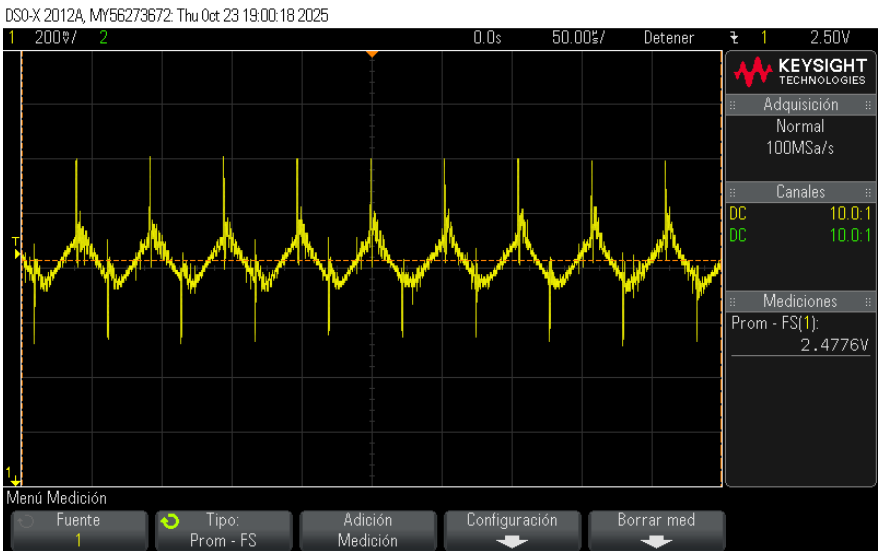
Figura 53: Corriente por el capacitor de salida.
