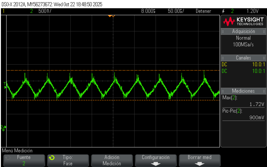
Figura 52: Corriente por el inductor.
