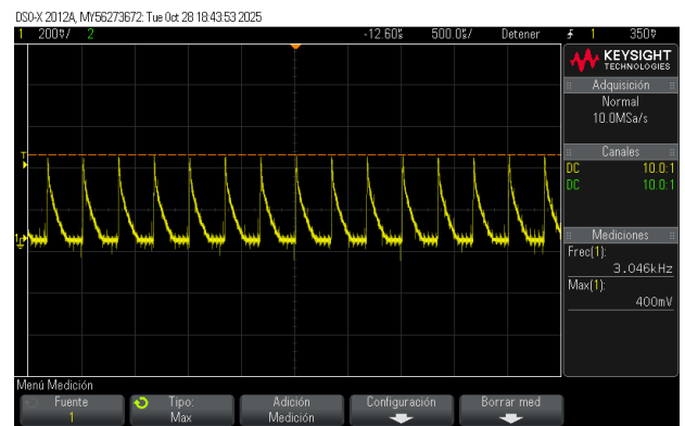
(b) Modo discontinuo de conducción (DCM).
