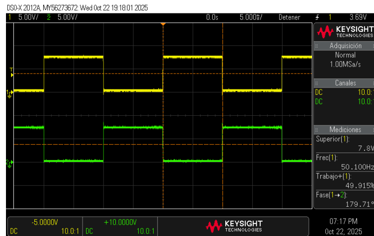
Figura 65: Tensión drenador-surtidor de los MOSFETs. En amarillo, Q1 y en verde, Q2.
