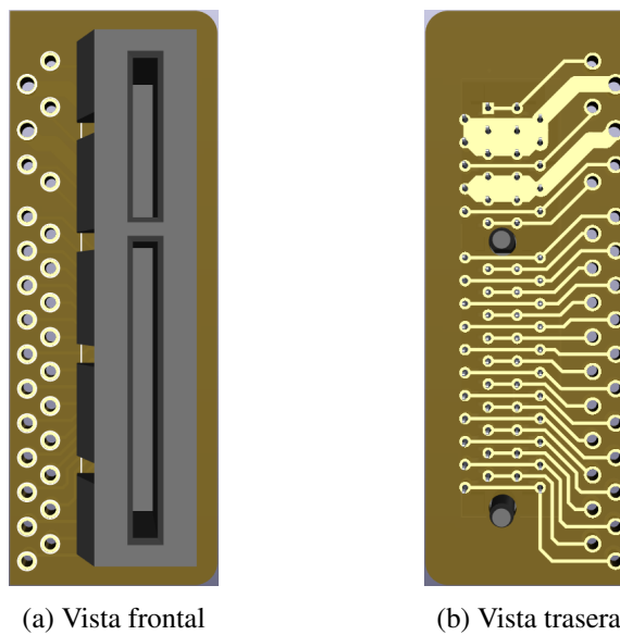
Figura 46: Modelo 3D de la mini-PCB para el conector PCIe x4.
