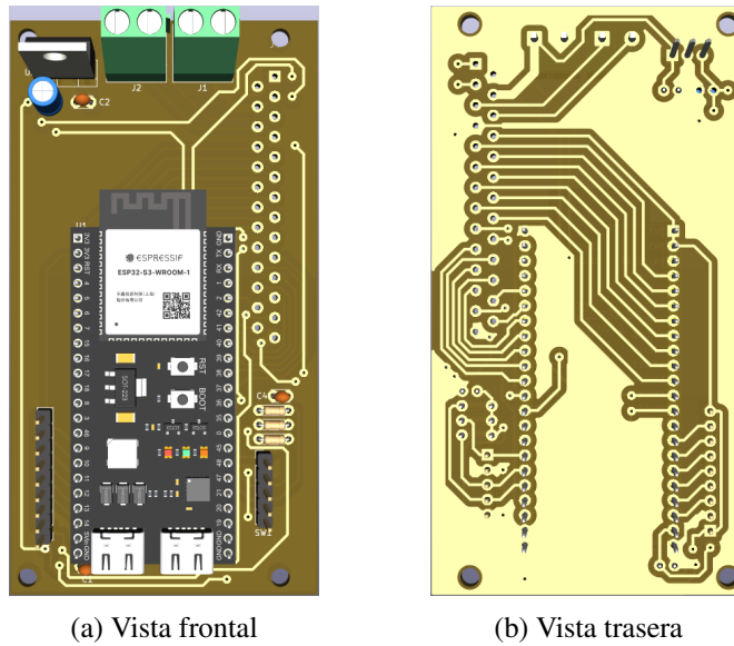
Figura 45: Modelo 3D de las PCB general del control del gabinete.
