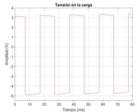
(b) Señal en la carga.
