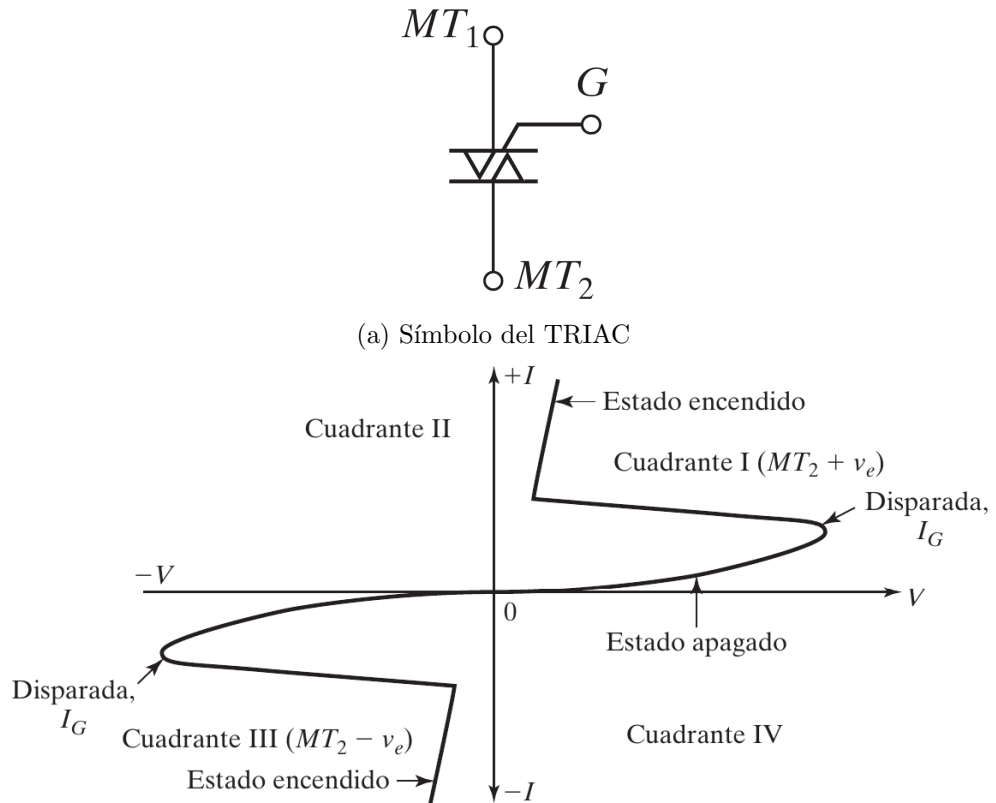
Figura 24: Características del TRIAC.
