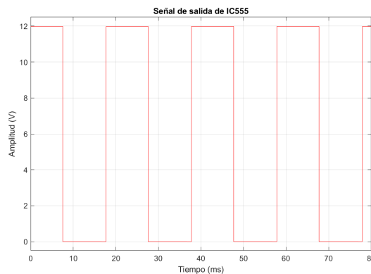
(a) Señal a la salida del IC555.
