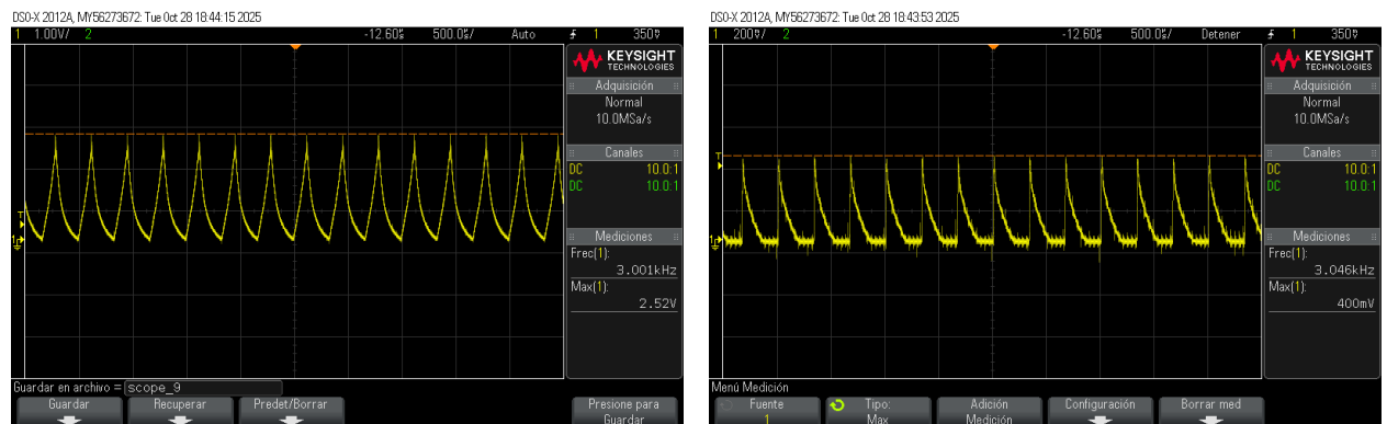
(a) Modo de conducción continua (CCM).
