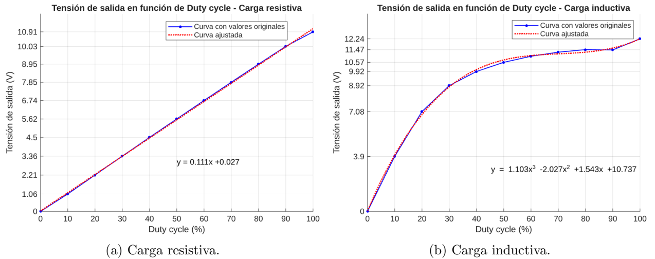
Figura 56: Tensión de salida del convertidor en función del PWM entregado por el microcontrolador, según tipo de carga.
