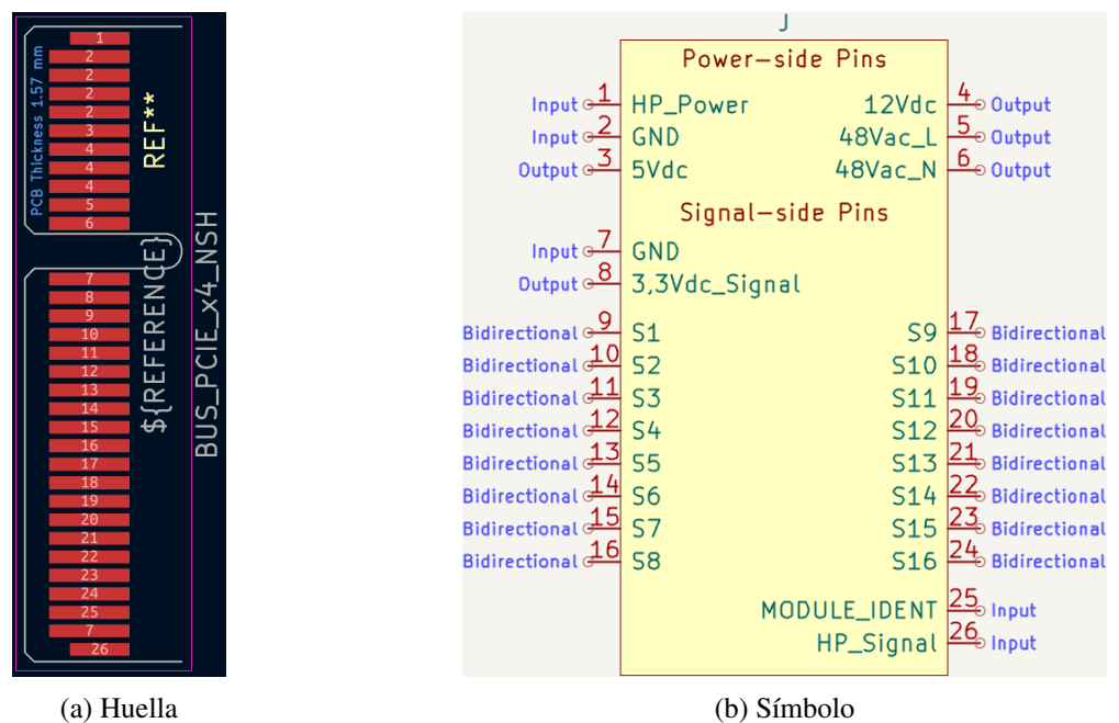
Figura 43: Símbolo y huella del conector PCIe x4
