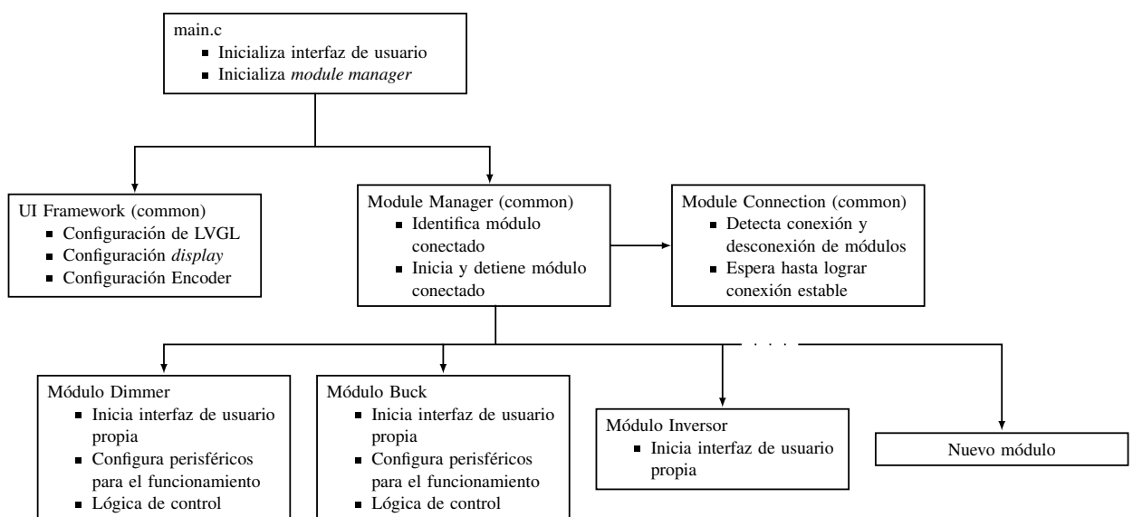
Figura 46: Estructura del código implementado
