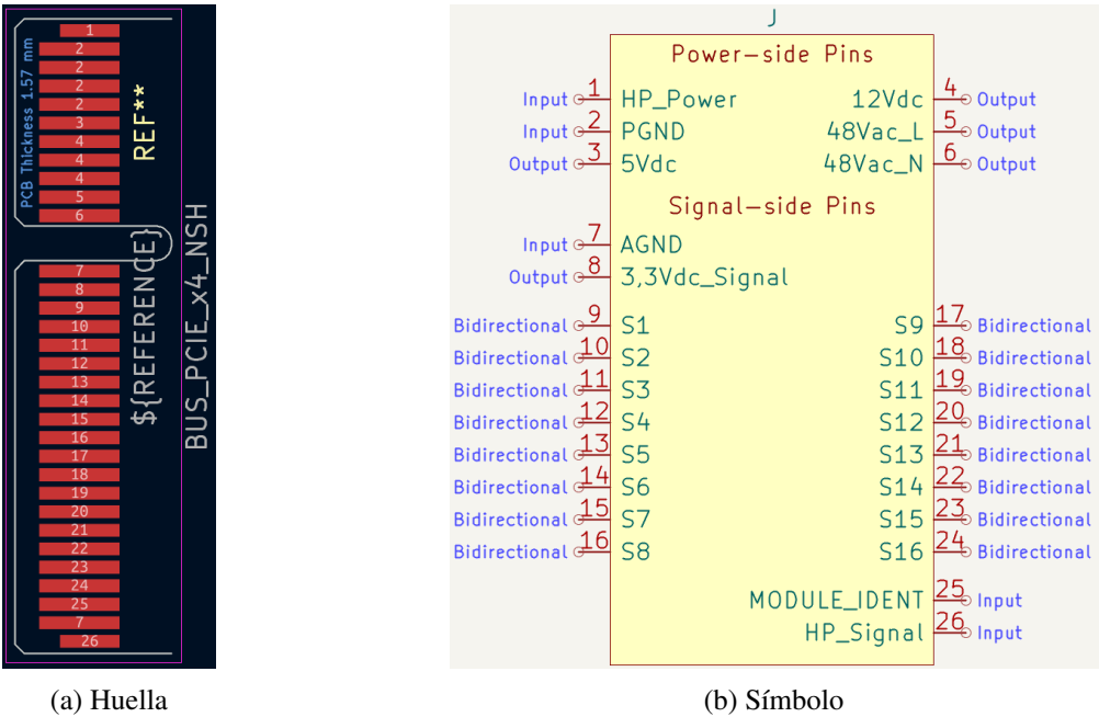
Figura 36: Símbolo y huella del conector PCIe x4
