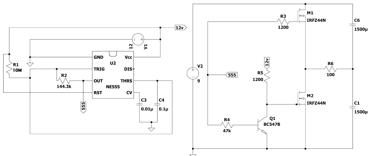
Figura 33: Circuito en LTSpice.
