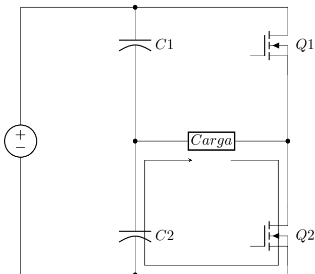
Figura 30: Conmutación 2.
