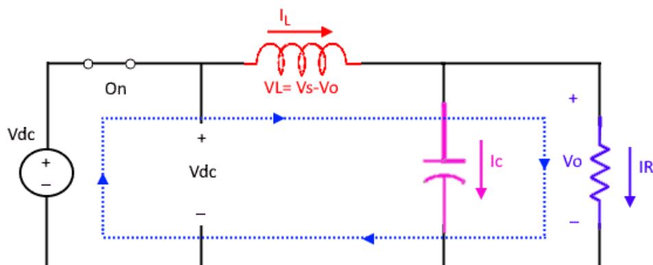
Figura 4: Interruptor en conducción.
