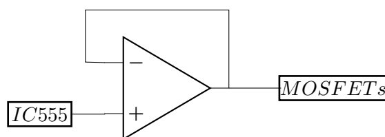
Figura 28: Seguidor de tensión.
