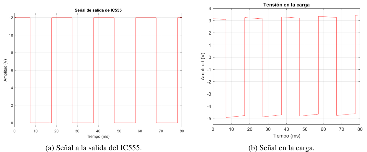
Figura 36: Gráficos de simulación
