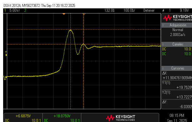
(b) Con capacitor de 400 pF.
