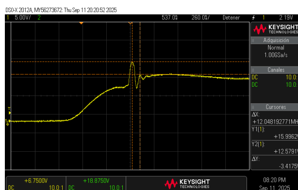
(b) Con capacitor de 2 pF 1 .
