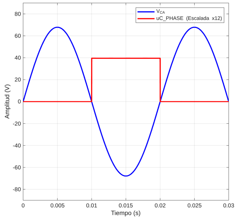
Figura 22: Entrada y salida del detector de cruce por cero (ZCD).
