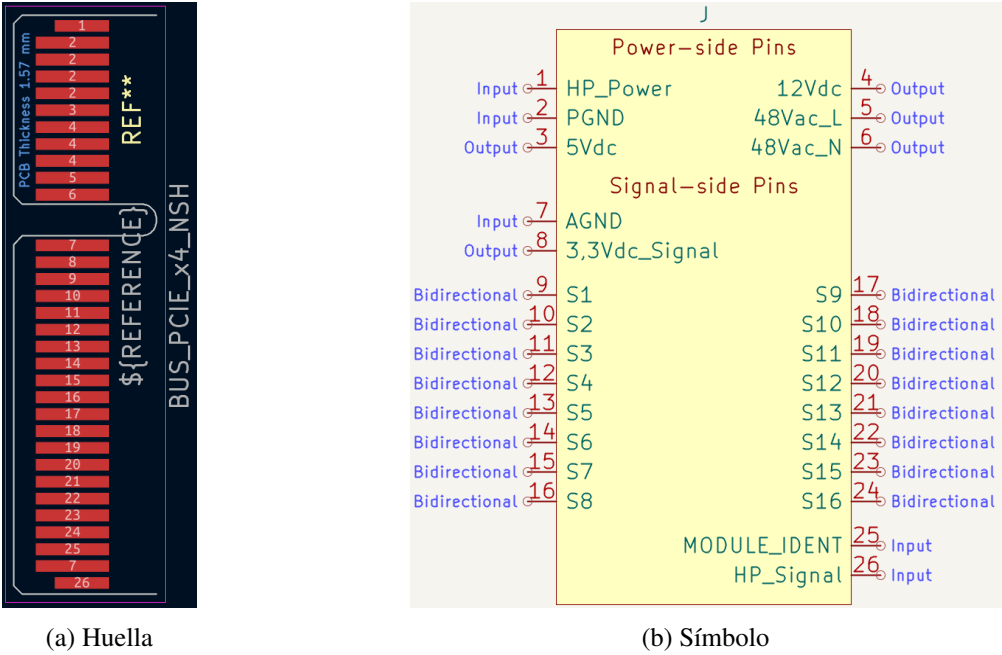
Figura 38: Símbolo y huella del conector PCIe x4
