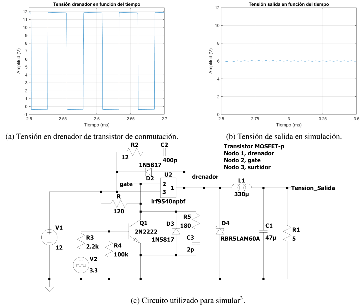
Figura 16: Resultados de la simulación con un ciclo de trabajo del 50 %.
