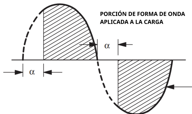
Figura 25: Control de fase de onda de corriente alterna. Fuente: (ON Semiconductor, 2005)
