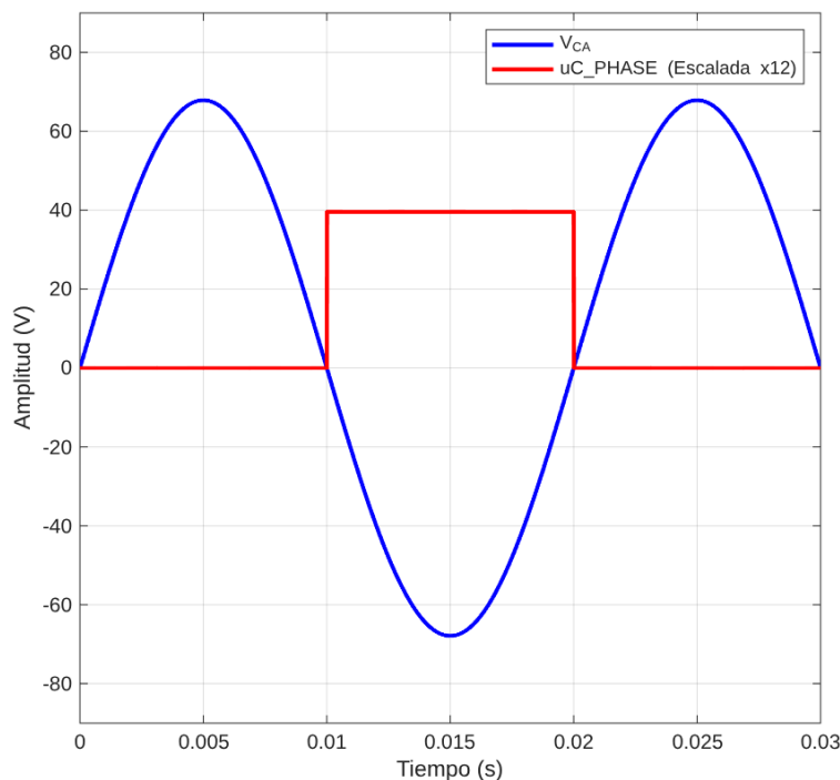
Figura 20: Entrada y salida del detector de cruce por cero (ZCD).
