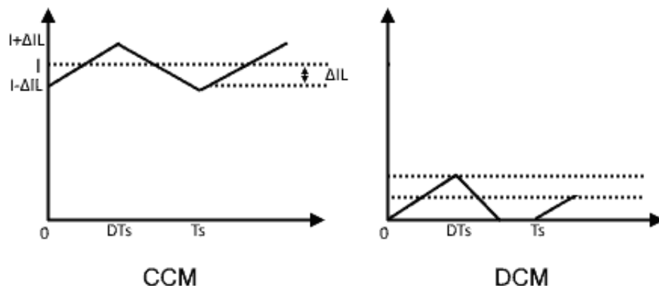
Figura 3: Modos de funcionamiento. Gentileza de Electrical Technology (Electrical Technology 2020, septiembre).
