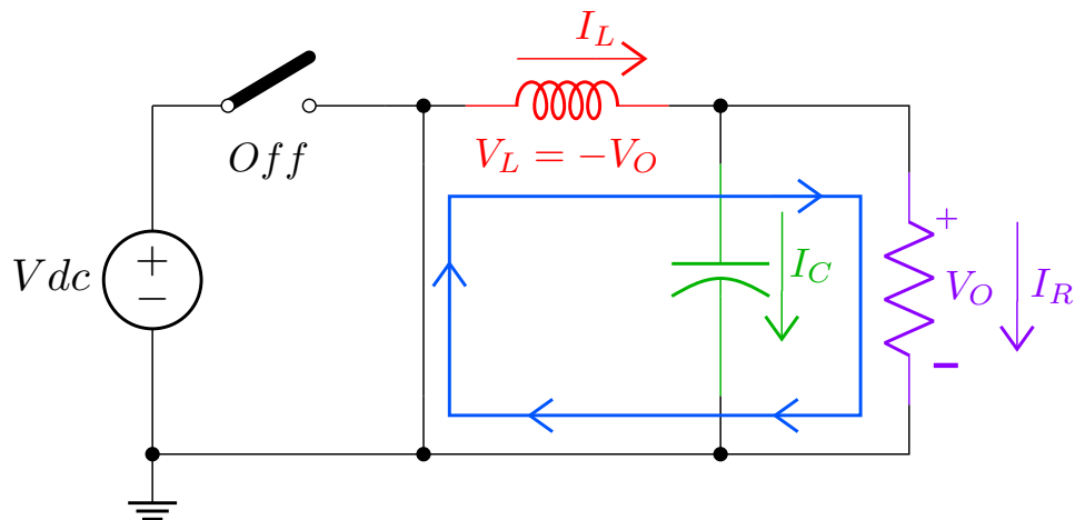
Figura 6: Interruptor en estado de no conducción.
