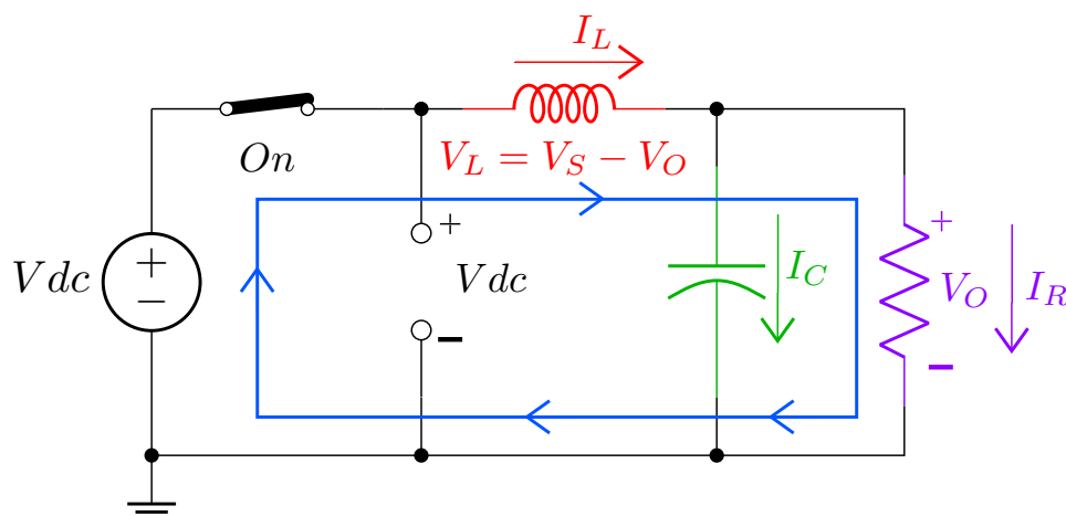
Figura 4: Interruptor en conducción.
