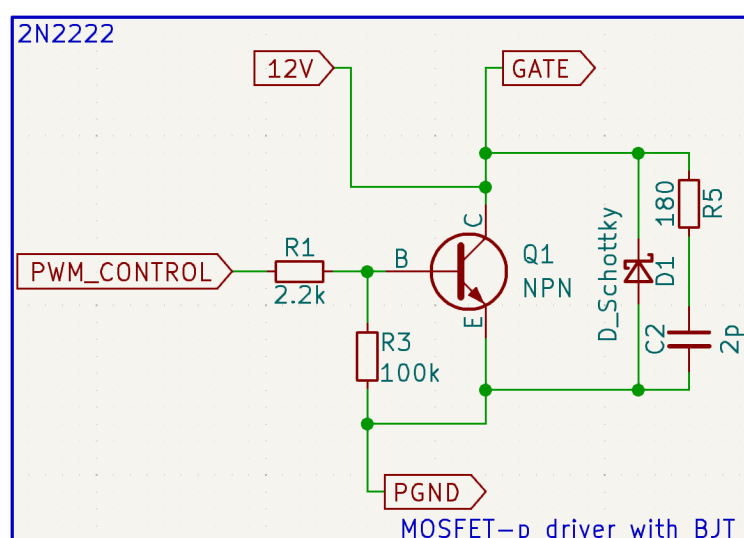
Figura 9: Transistor 2N2222 como driver de MOSFET-p.
