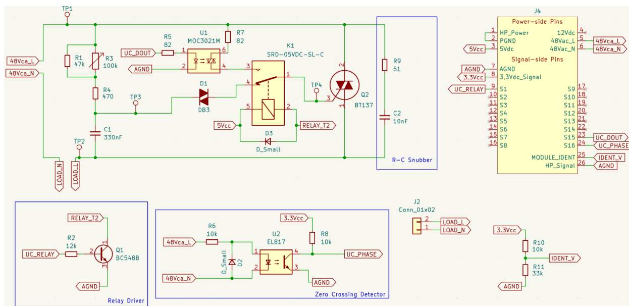
Figura 9: Circuito completo del módulo recortador de onda.
