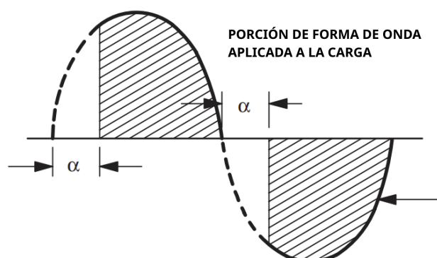
Figura 2: Control de fase de onda de corriente alterna. REFERENCIA Thyristor Theory and Design Considerations
