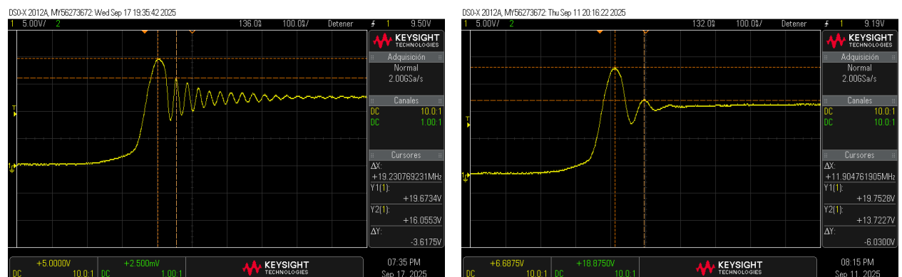
(a) Sin capacitor.
