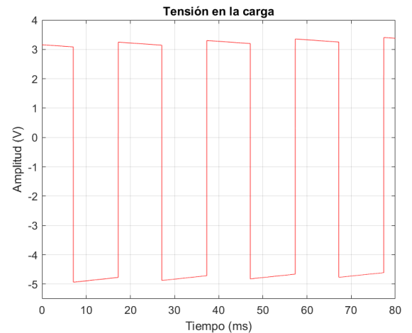
(b) Señal en la carga.
