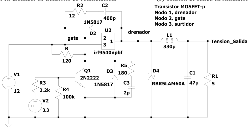
(c) Circuito utilizado para simular 3 .
