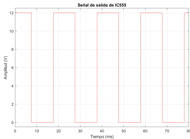
(a) Señal a la salida del IC555.
