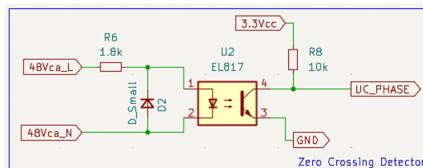
Figura 6: Circuito ZCD.
