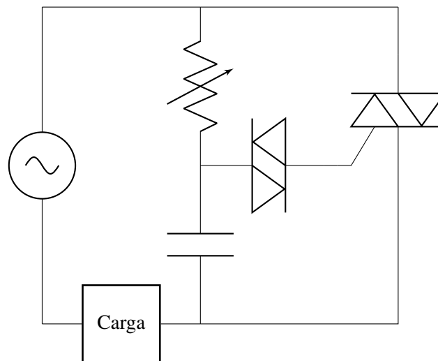
Figura 1: Circuito básico recortador de onda analógico.
