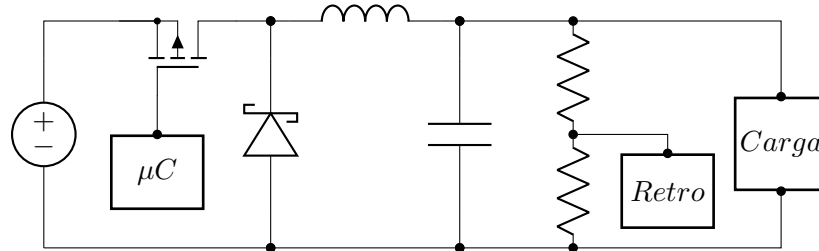
Figura 1: Circuito básico del convertidor Buck.
