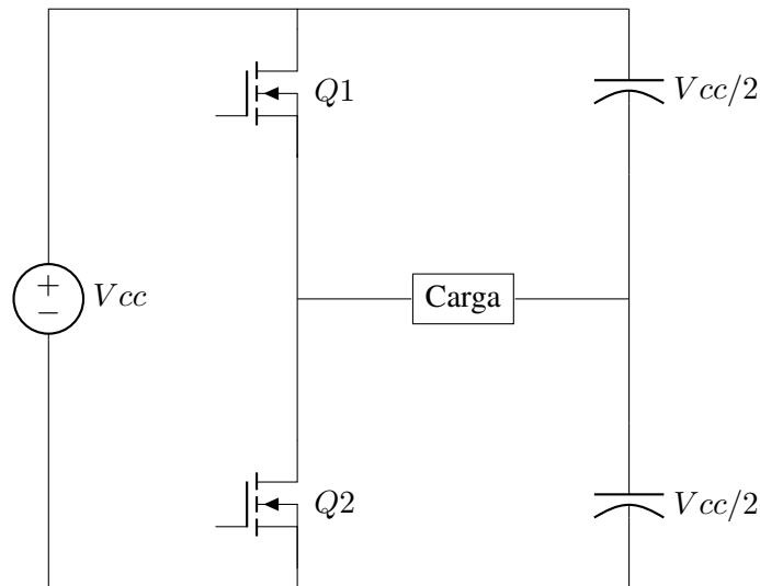
Figura 28: Inversor medio puente con control por 555
